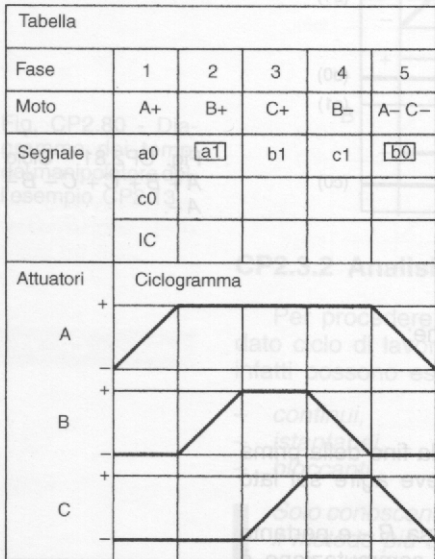
Fig. CP2.83 - Ciclo A+ B+ C+ B- (A- C-).
