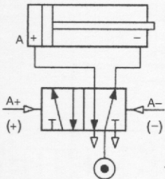
Fig. CP2.65 - Convenzione sui distributori di potenza.
