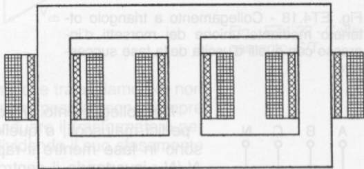
Fig. ET4.15 - Trasformatore trifase a tre colonne complanari.
