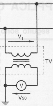
Fig. ET4.25 - Trasformatore di misura TV.
