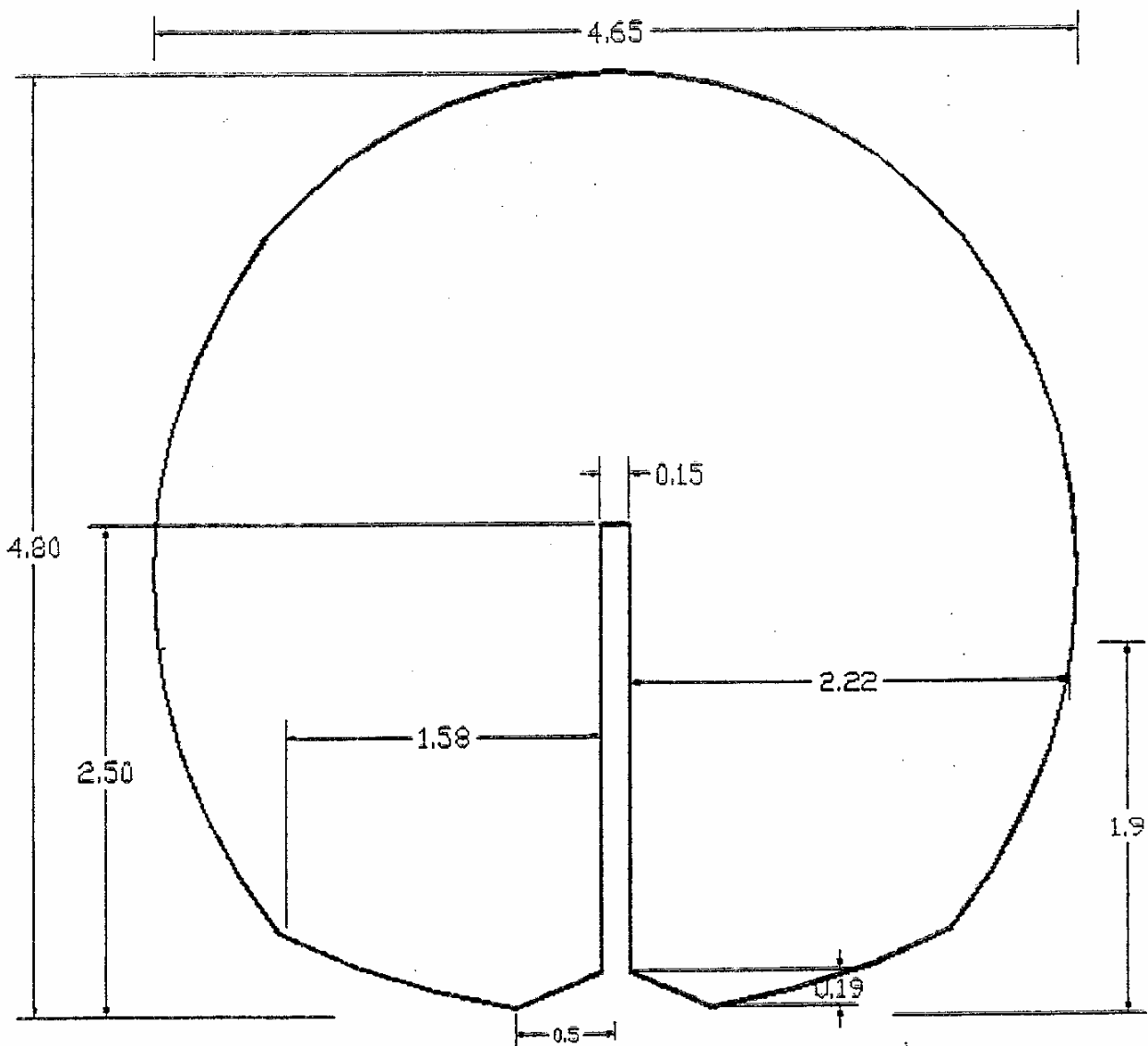
galleria ex-Casmez modificata
