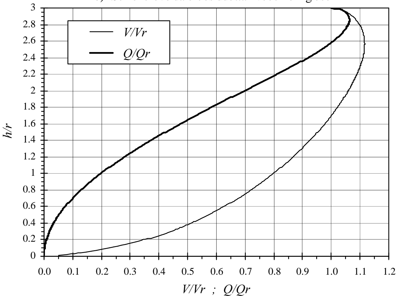
b) Sezione ovoidale cosiddetta "vecchio inglese"
