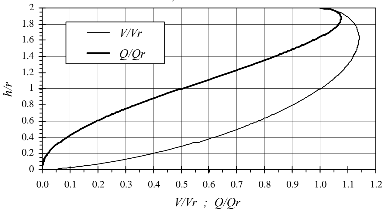
a) Sezione circolare
