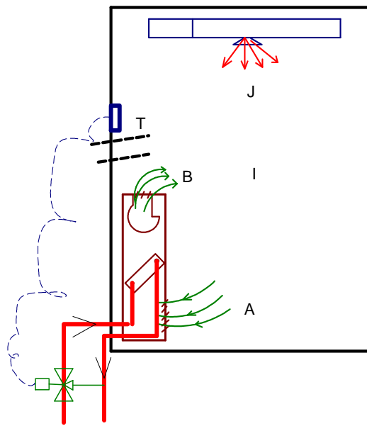
Figura 280: Regolazione dei fan coil mediante valvola a tre vie
