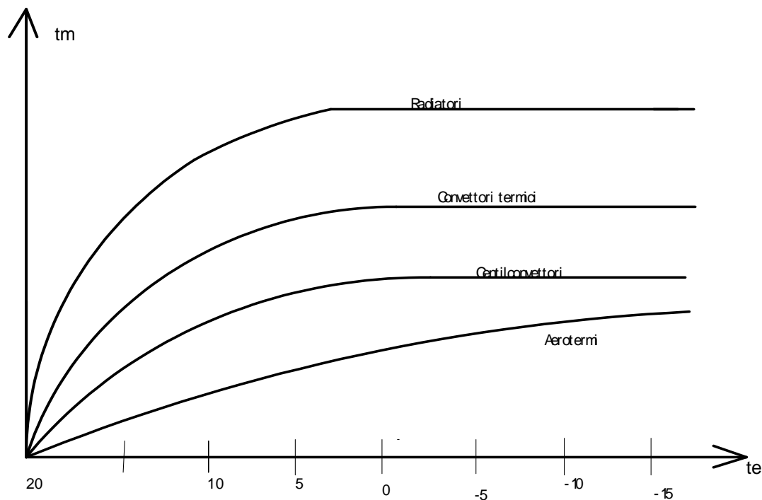
Figura 331: Curve di regolazione delle centraline
