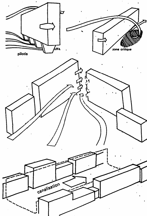
Figura 195: Effetti di canalizzazione e Venturi provocati dagli edifici
