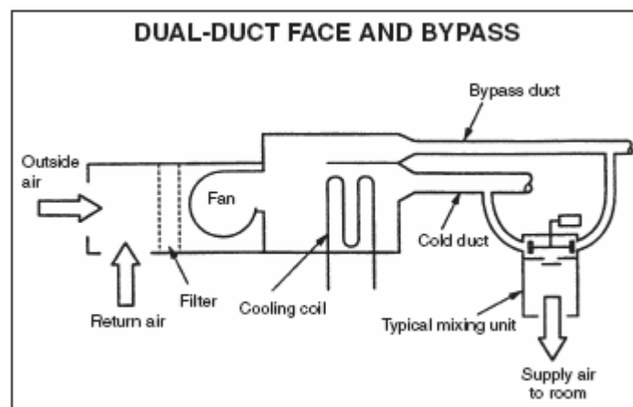
Figura 355: Controllo mediante doppio condotto
