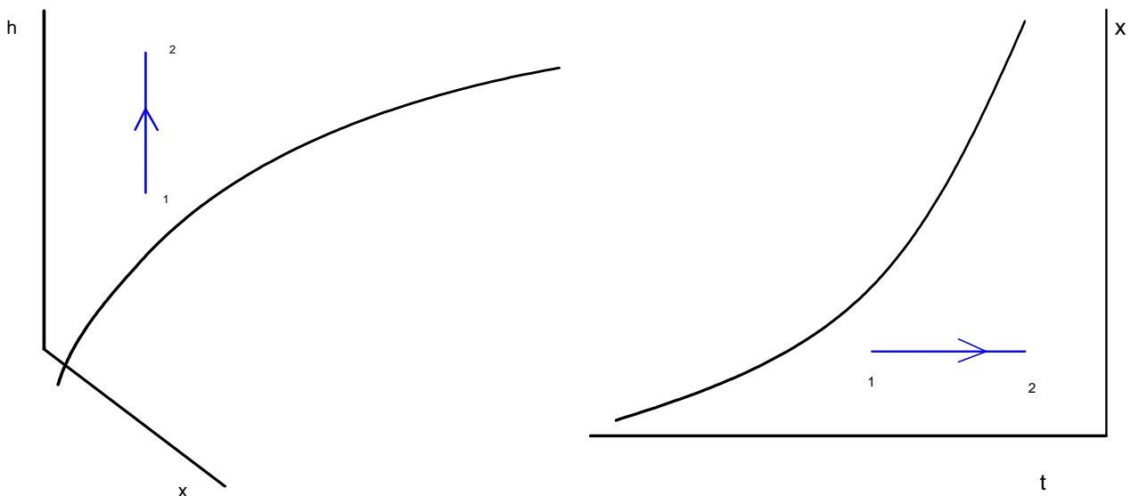
Figura 218: Riscaldamento sensibile nel piano di Mollier ed ASHRAE
