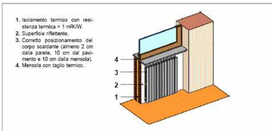
Figura 157: Corretta installazione di un radiatore
