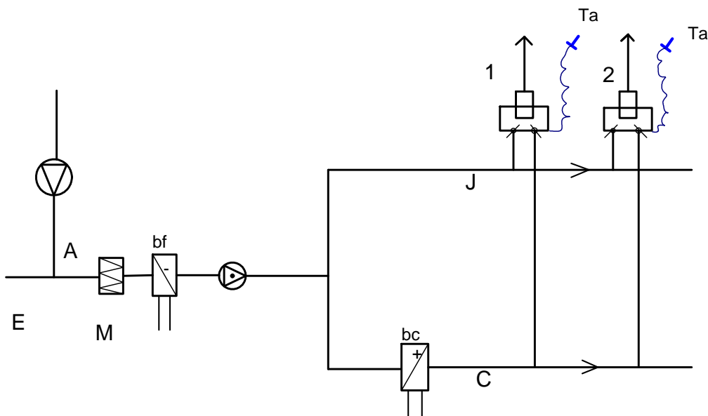
Figura 258: Schema alternativo per impianto dual conduit estivo
