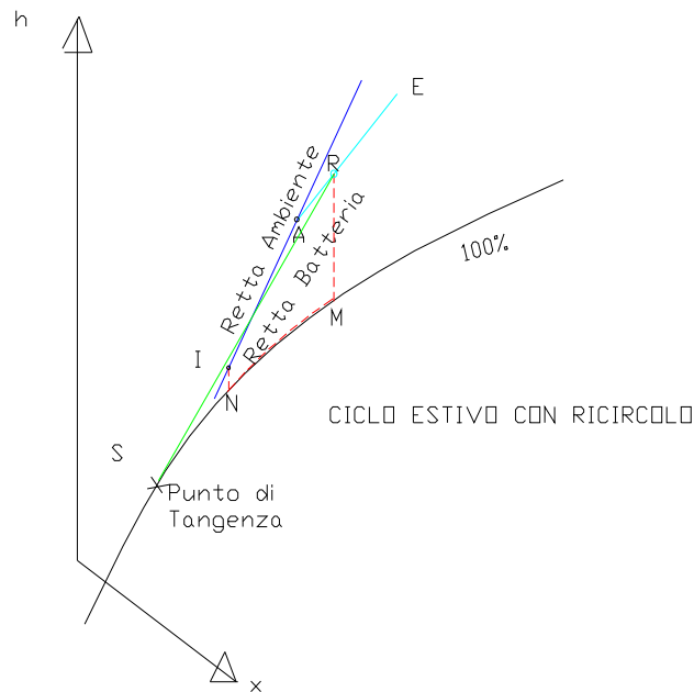
Figura 242: Ciclo estivo con ricircolo
