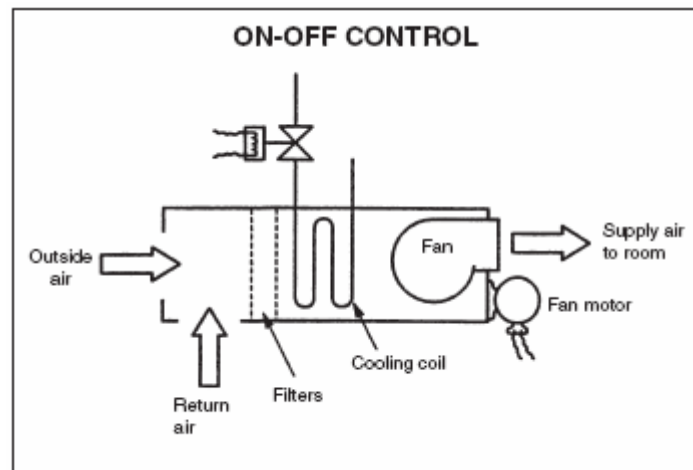
Figura 349: Sistema di controllo On-Off
