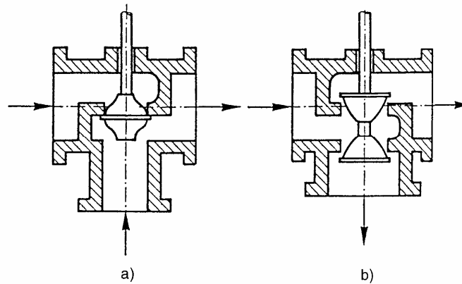
Figura 308: Tipologie di valvole a tre vie: Miscelatrici e Deviatrici
