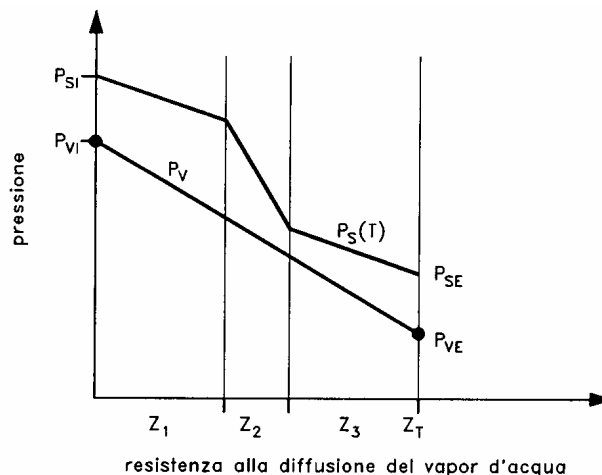
Figura 127: Diagramma di Glaser per le pressioni parziali di vapore
