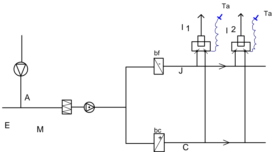
Figura 256: Impianto Dual Conduit in regime estivo
