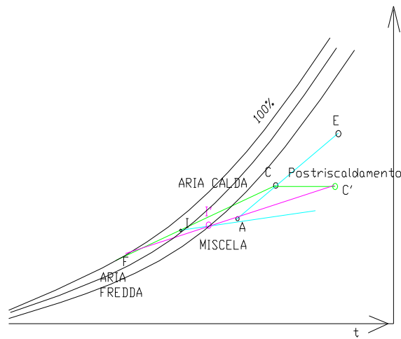
Figura 254: Miscelazione dell'aria in un impianto a doppio canale
