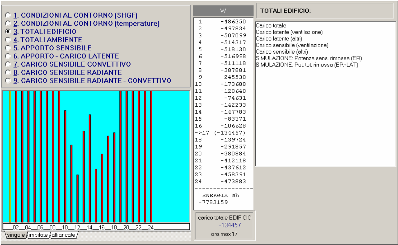
Figura 175: Carico orario del mese di gennaio per l'intero edificio protetto con film riflettente
