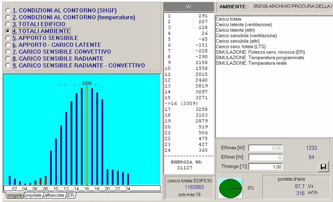
Figura 174: Carico termico orario per il 21 giugno in un ambiente a NW al 2° piano edificio originale
