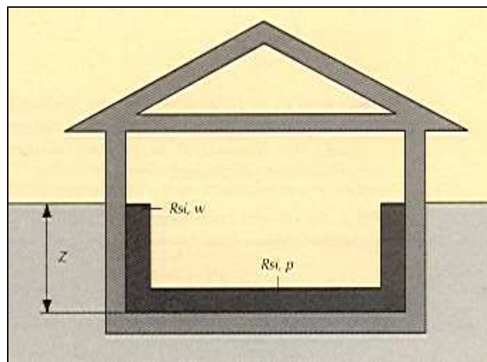
Figura 148: Scambi termici con piano interrato.
