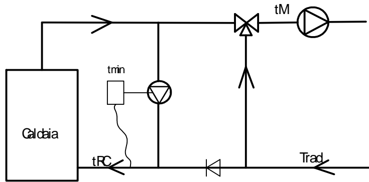
Figura 336: Caldaia con valvola a tre vie e ricircolo
