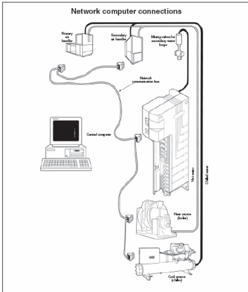
Figura 320: Collegamenti del controller locale ai dispositivi e al computer centrale
