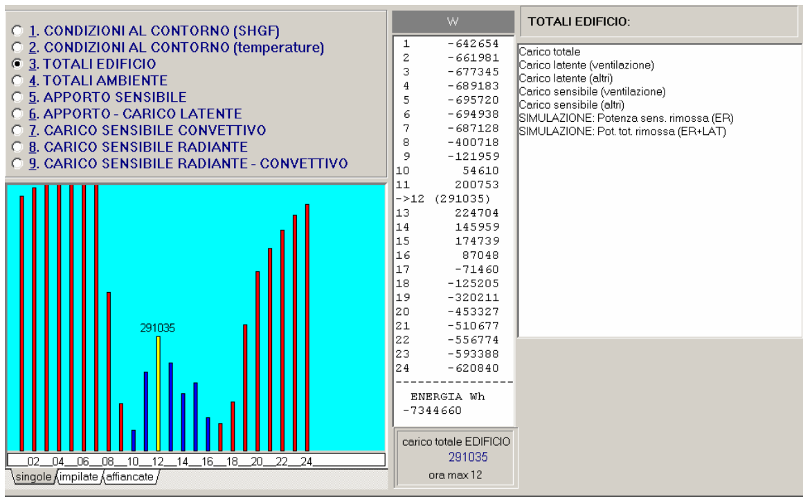
Figura 167: Andamento orario del carico termico nel mese di gennaio per edificio originale
