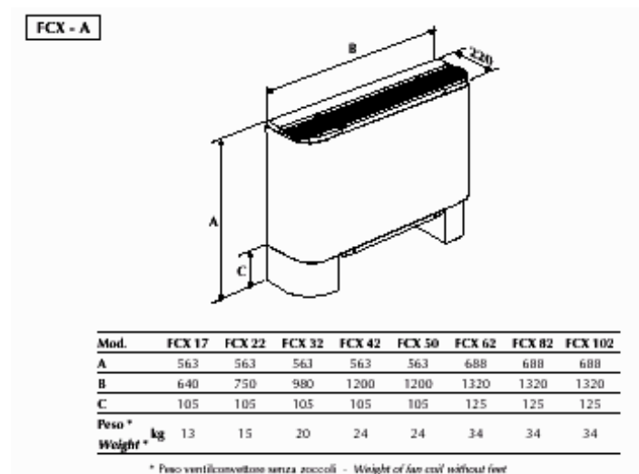
Figura 272: Dati dimensionali dei fan coil
