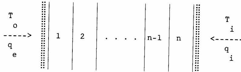
Figura 44: Parete multistrato con scambio termico
