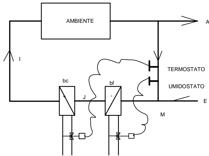
Figura 347: Schema di regolazione con batteria di post riscaldamento
