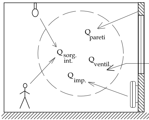
Figura 47: Bilancio energetico per l'aria interna all'ambiente
