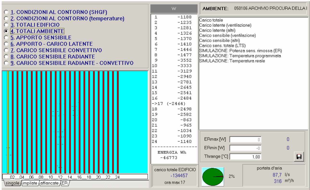
Figura 177: Carichi orari per un ambiente a NW al 2° piano per edificio protetto con film
