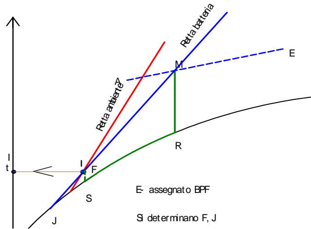
Figura 238: Retta ambiente interseca la curva di saturazione: caso B
