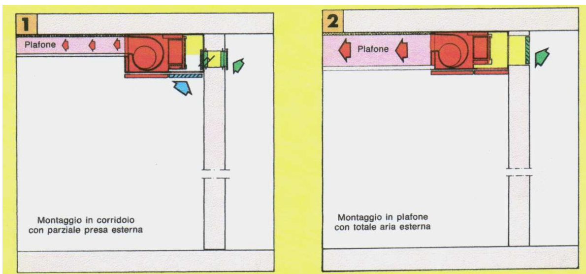
Figura 288: Disposizione dei fan coil canalizzati
