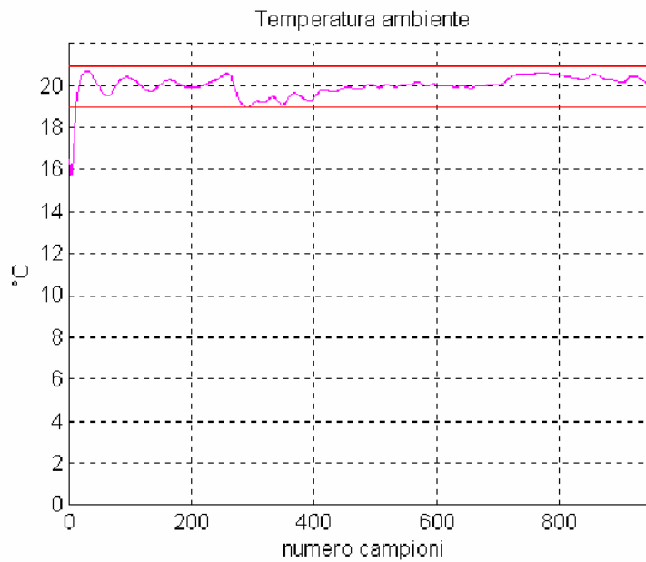
Figura 293: Andamento della temperatura ambiente termostata
