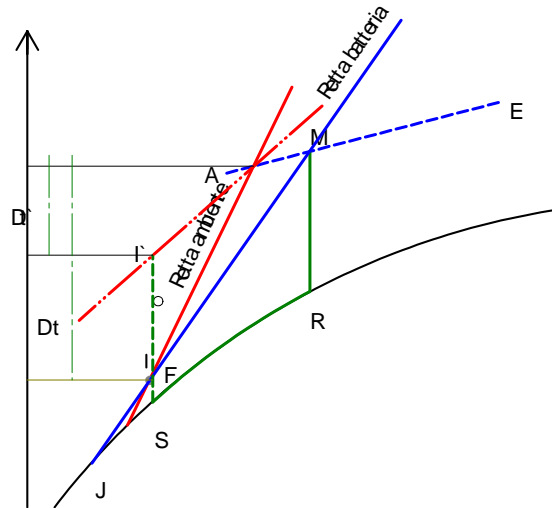
Figura 346: Regolazione del carico sensibile con batteria di postriscaldamento
