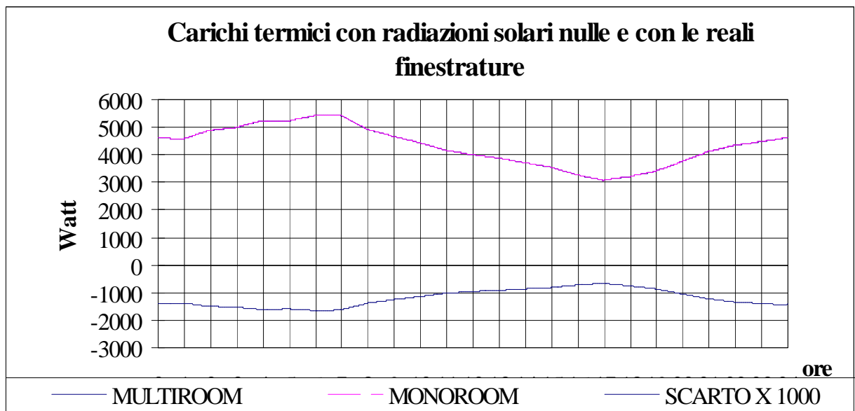
Figura 52: Andamento dei carichi termici con finestrate
