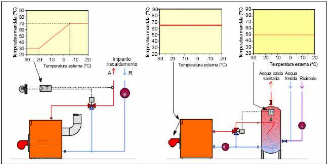
Figura 163: Generatori separati per riscaldamento e produzione di acqua calda sanitaria
