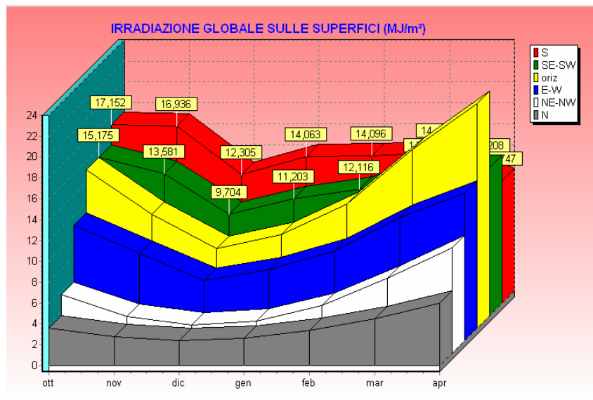
Figura 168: Andamento della radiazione solare per il mese di gennaio per il sito di progetto
