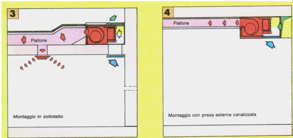
Figura 289: Disposizione dei fan coil canalizzati
