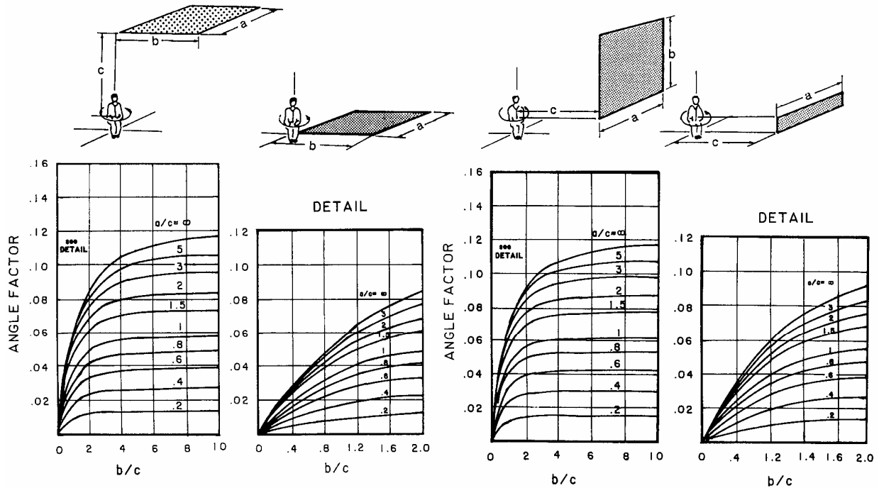
Figura 18: Fattori di vista fra corpo umano e pareti verticali ed orizzontali (Fanger 1982)
