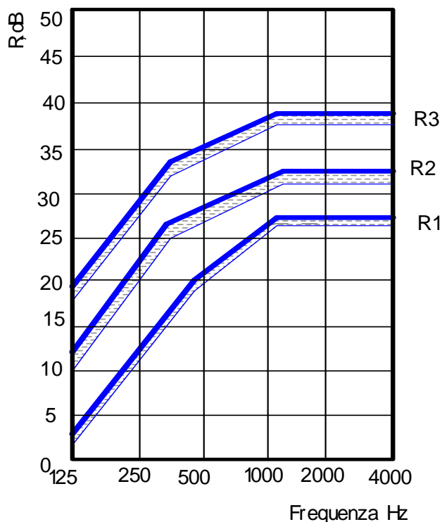
Figura 39: Classificazione acustica degli infissi
