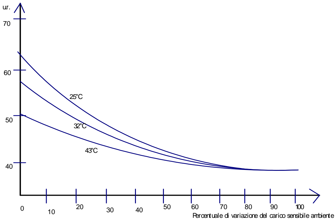
Figura 263: andamento dell'umidità relativa al variare del carico sensibile
