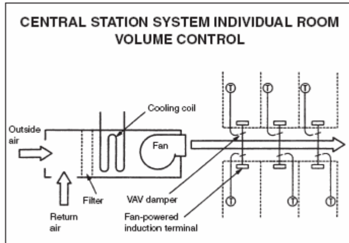
Figura 353: Controllo a portata d'aria variabile (VAV)
