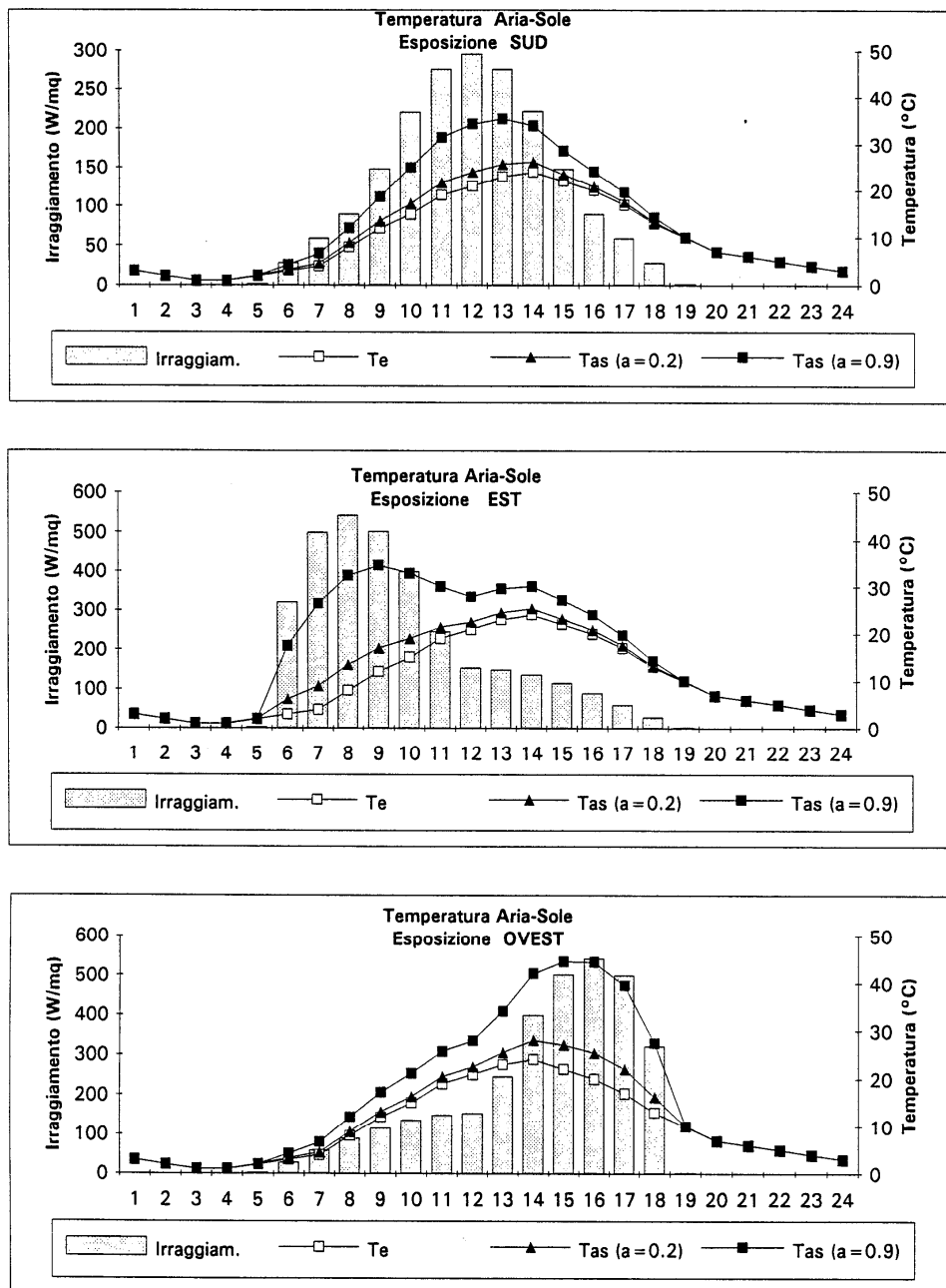
Figura 37: Temperatura aria-sole per a=0.2 e a=0.9 ed esposizione Sud, Est ed Ovest.
