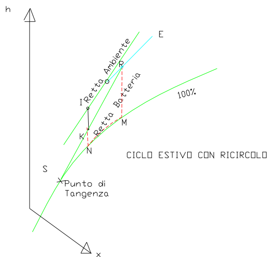
Figura 243: Ciclo estivo con ricircolo e postriscaldamento
