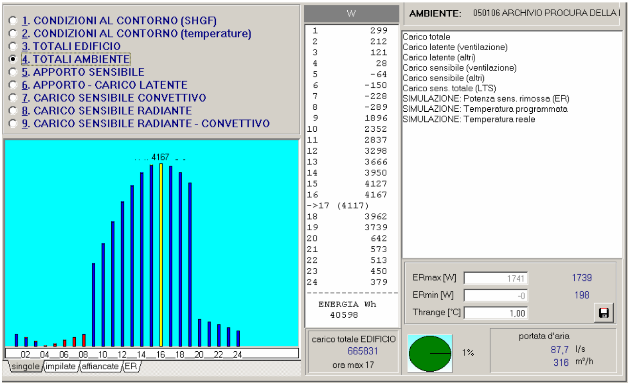
Figura 180: Carichi in giugno orari per l'ambiente a NW a 2° piano con edificio con film riflettente
