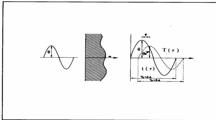
Figura 29: Trasmissione del calore in uno strato seminfinito: risposta alla forzante esterna sinusoidale.
