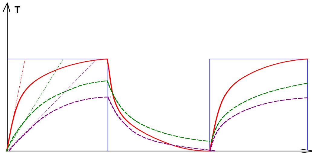
Figura 33: Transitorio termico con diverse costanti di tempo
