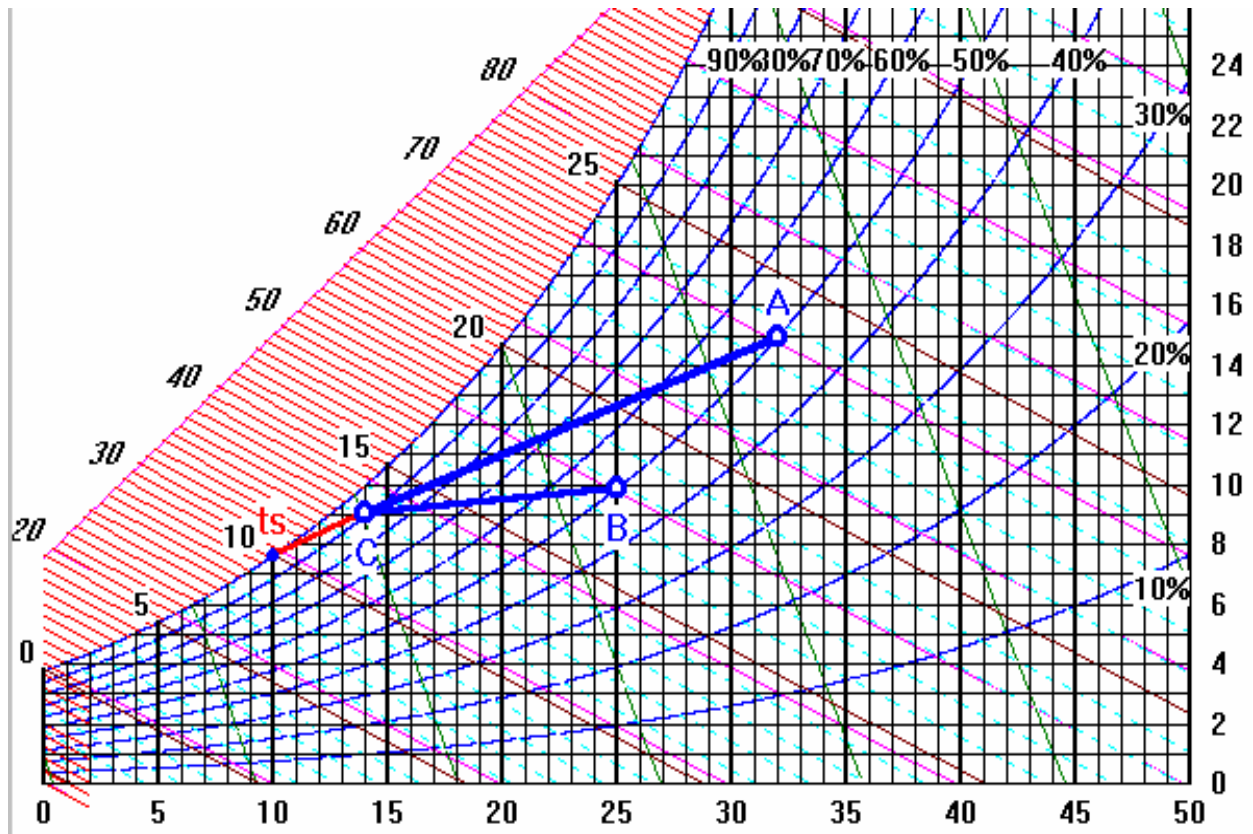
Figura 233: Ciclo estivo con deumidificazione nel piano ASHRAE
