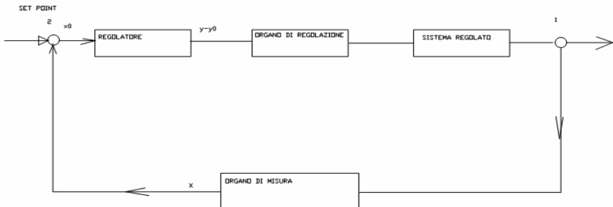
Figura 303: Schema di regolazione chiuso a feedback
