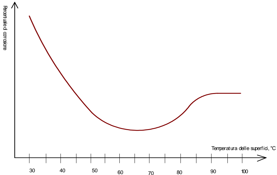
Figura 333: Velocità di corrosione in funzione delle temperatura superficiale
