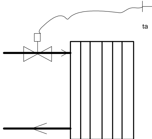
Figura 339: Schema di applicazione di una valvola termostatica sul radiatore
