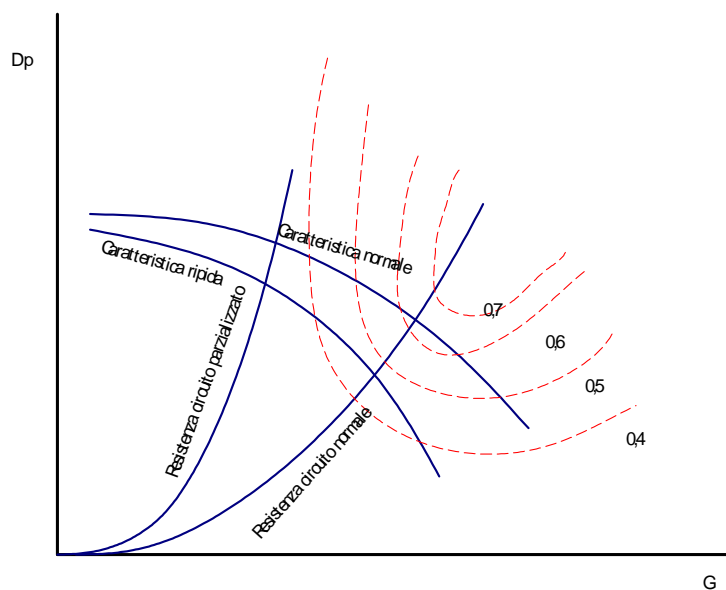
Figura 342: Spostamento del punto di lavoro per effetto della parzializzazione
