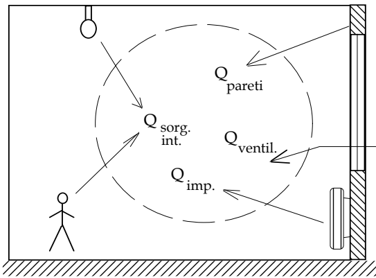
Figura 41: Bilancio energetico per l'aria interna all'ambiente
