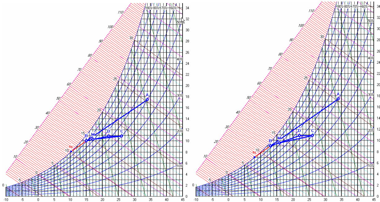
Figura 282: Relazione estiva mediante variazione delle condizioni dell'aria primaria
