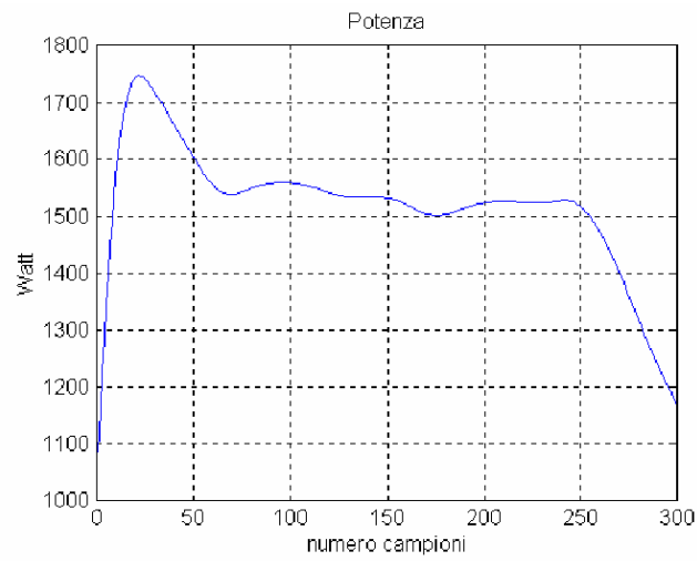
Figura 296: Andamento della potenza ceduta prevista dal controller neurale
