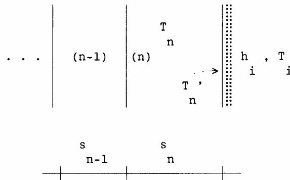
Figura 46: Schematizzazione della parete multistrato
