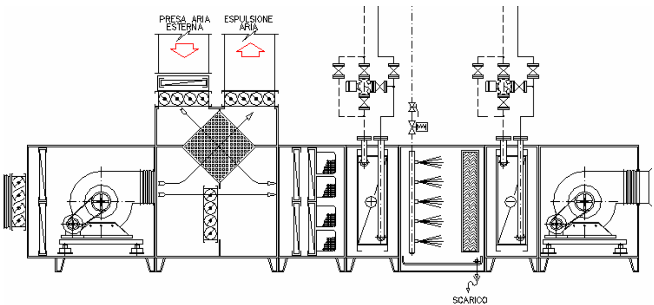
Figura 231: Centrale di Trattamento Aria con ricircolo e recuperatore di calore
