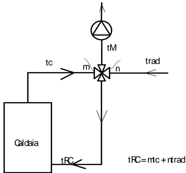
Figura 336: Caldaia con valvola a tre vie e ricircolo
