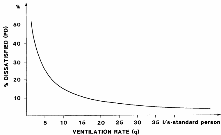
Figura 25: Correlazione sperimentale fra PPD e Portata d'aria di ventilazione
