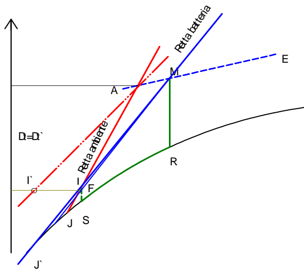
Figura 348: Regolazione del carico latente con batteria di postriscaldamento
