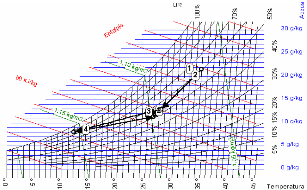
Figura 247: Ciclo estivo con ricircolo nel piano ASHRAE
