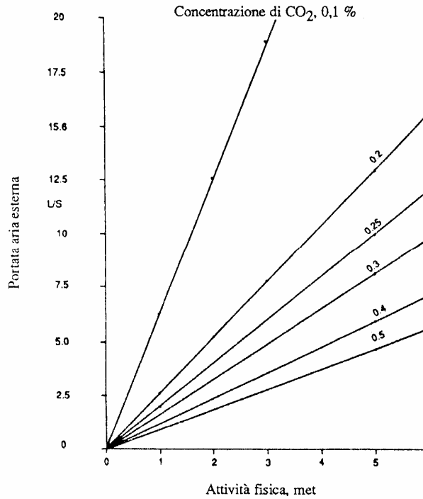
Figura 21: Portata di aria esterna al variare dell'attività fisica e della % di CO 2
