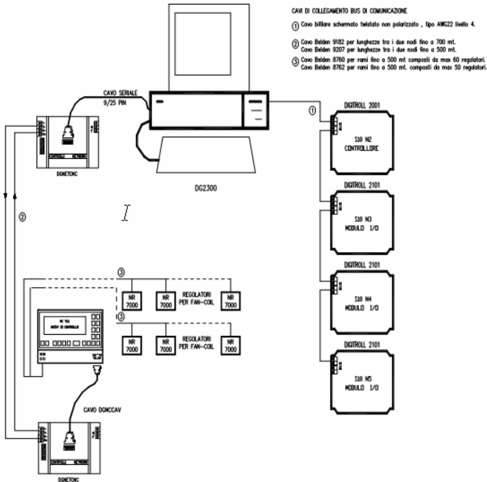
Figura 310: Sistema di controllo centralizzato mediante computer
