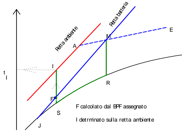
Figura 235: Retta ambiente non interseca la curva di saturazione: caso A
