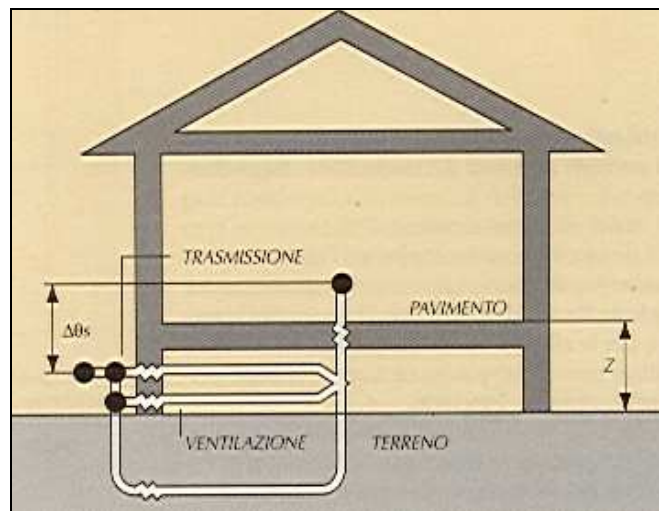
Figura 147: Trasmissione del calore con spazio aerato nel terreno
