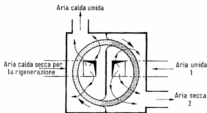
Figura 224: Schema di funzionamento di un deumidificatore igroscopico continuo
