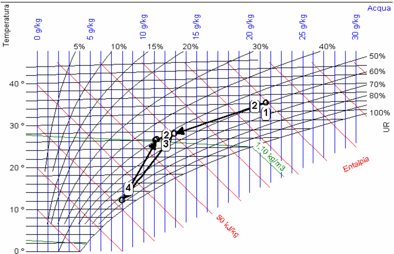
Figura 246: Ciclo estivo con ricircolo nel piano di Mollier
