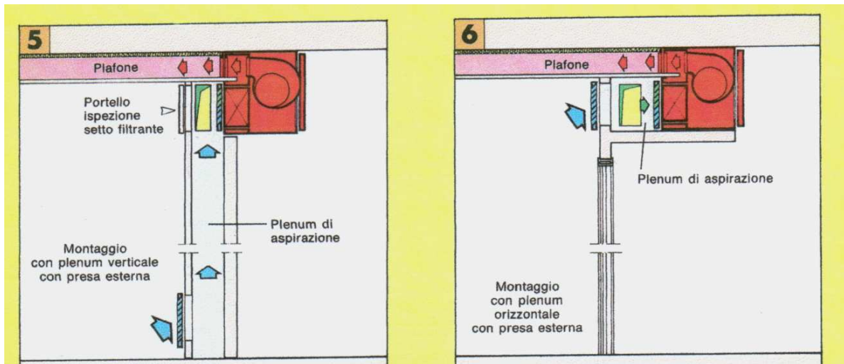
Figura 287: Disposizione dei fan coil canalizzati
