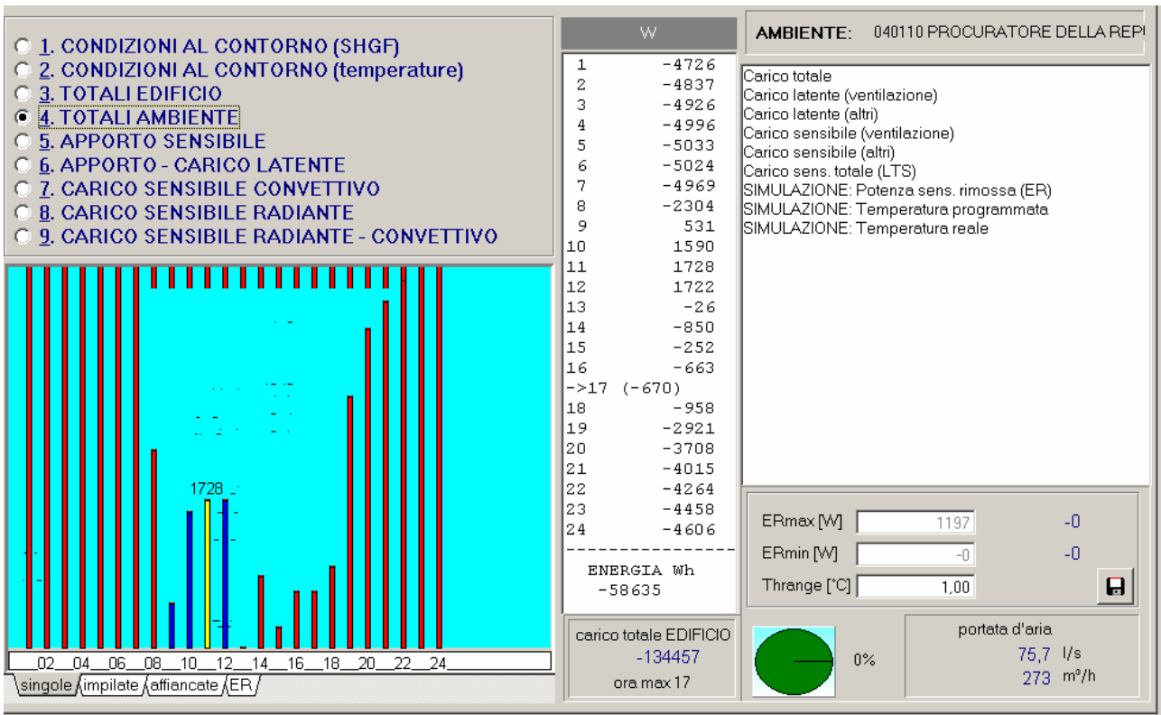
Figura 176: Carichi orari per un ambiente di riferimento a 2° piano per edificio protetto con film
