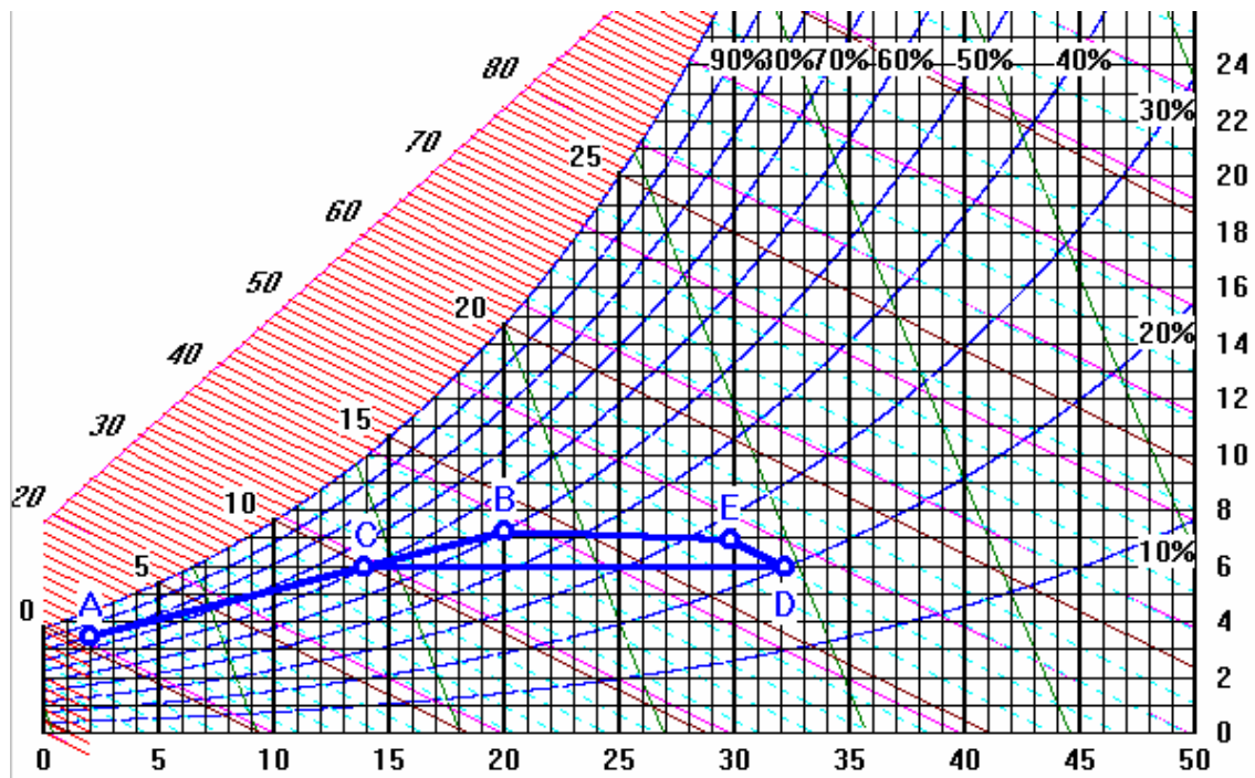
Figura 251: Ciclo di condizionamento invernale con ricircolo e parziale saturazione – ASHRAE
