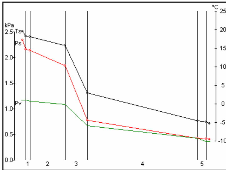
Figura 130: Esempio di verifica Glaser per la parete composta
