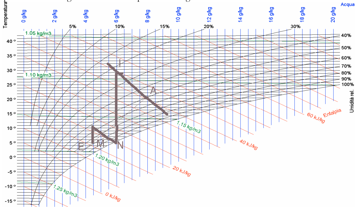
Diagramma di Mollier per aria umida - Pressione 0.950 bar (537.000 m / 10.000 °C / 80.000 % Ur)
