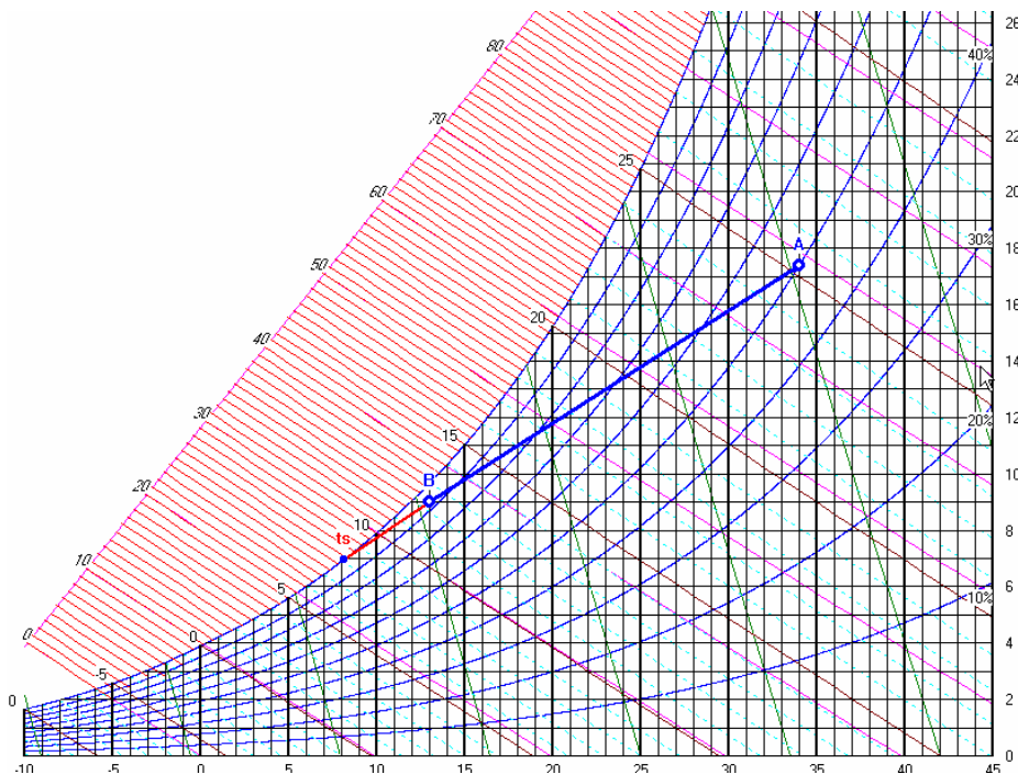
Figura 273: Trattamento aria primaria in condizioni estive
