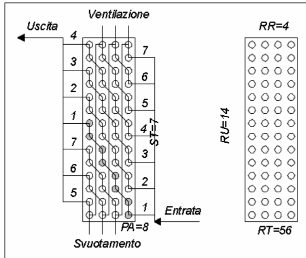
Figura 216: Passaggi del fluido interno nella batteria alettata
