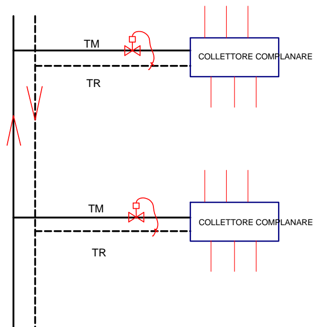
Figura 338: Schema di regolazione di zona
