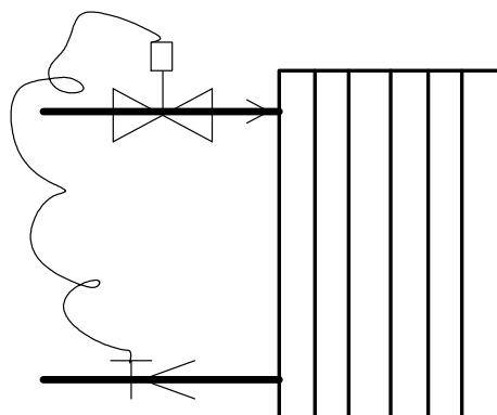
Figura 340: Valvola termostatica con controllo sul ritorno
