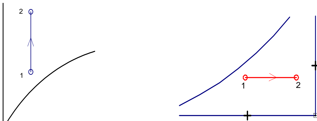
Figura 121: Rappresentazione del riscaldamento dell'aria umida.
