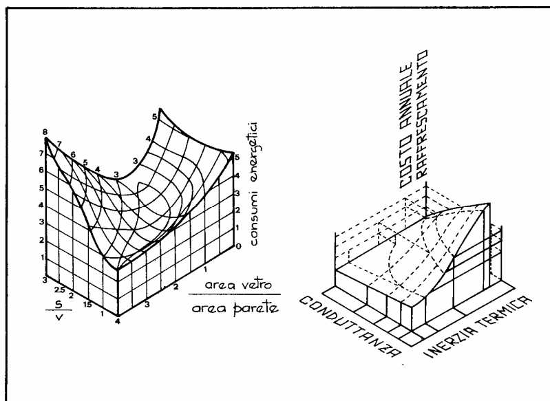
Figura 55: Consumi energetici di un edificio per riscaldamento e raffreddamento in funzione del rapporto Superficie disperdenti e volume ( S/V ) e del rapporto Sup. \text{ vetrata} - Sup. \text{ muraria} ( Sv/Sm ). Energia annualmente trasmessa da una parete in funzione della trasmittanza e dell'inerzia termica (fattore \gamma ).
