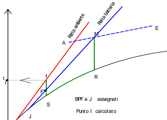
Figura 237: Retta ambiente interseca la curva di saturazione: caso A
