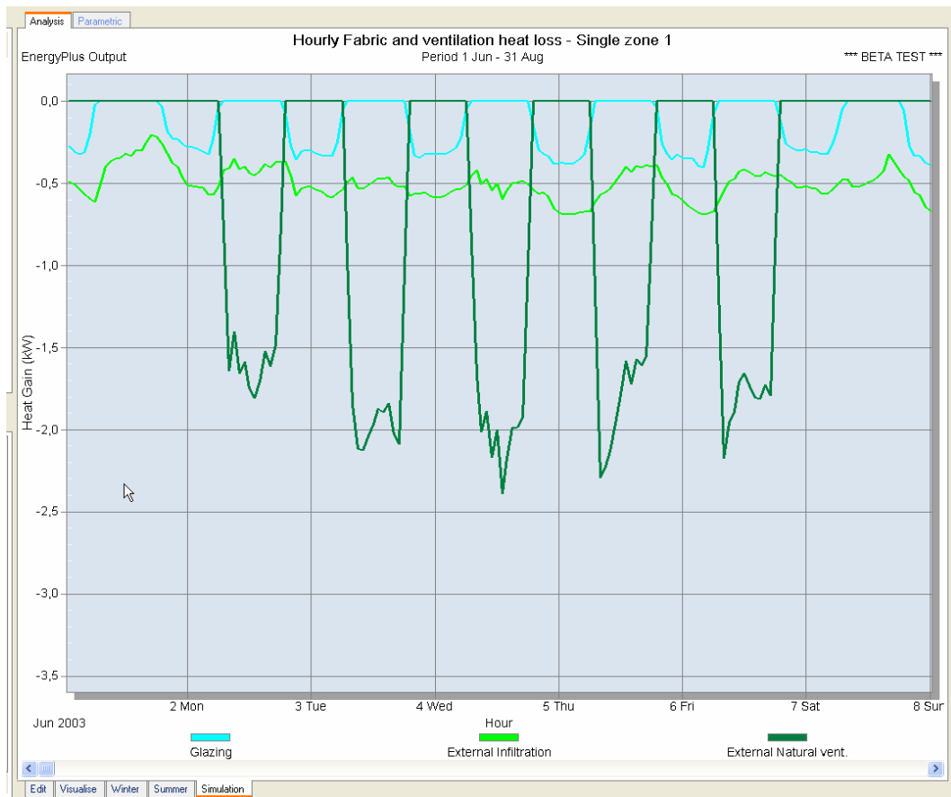
Figura 93: Visualizzazione delle perdite per ventilazione
