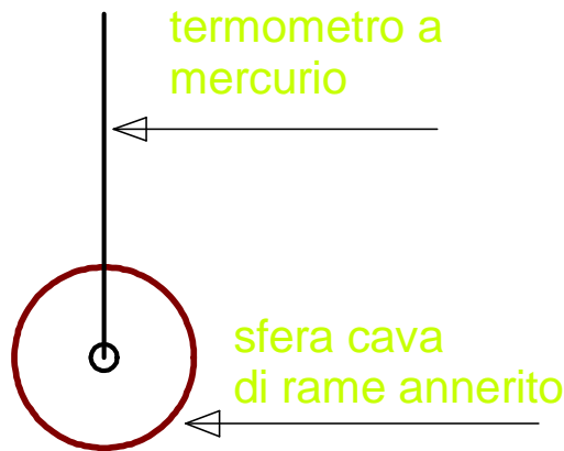
Figura 8: Schema del globotermometro di Bedford
