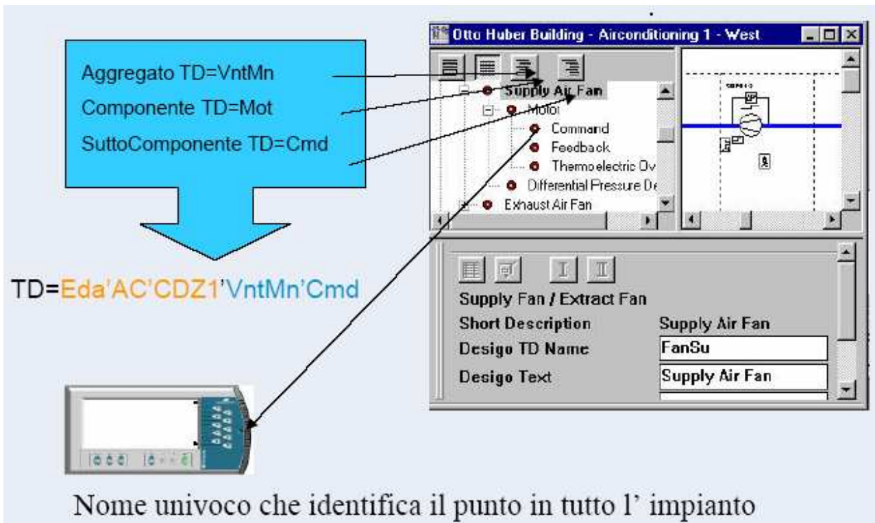
Figura 324: Esempio di programmazione dei controller locali
