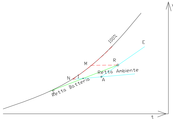
Figura 244: Ciclo estivo con ricircolo – ASHRAE
