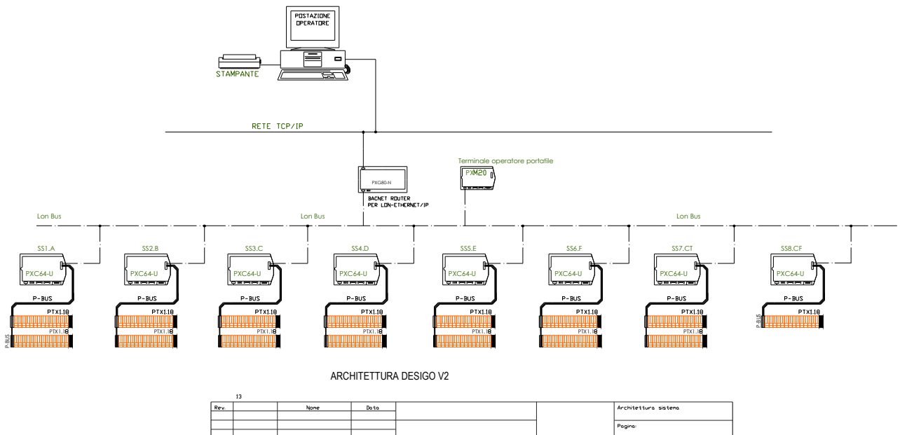
Figura 312: Esempio di controllo distribuito e bus di trasmissione dati
