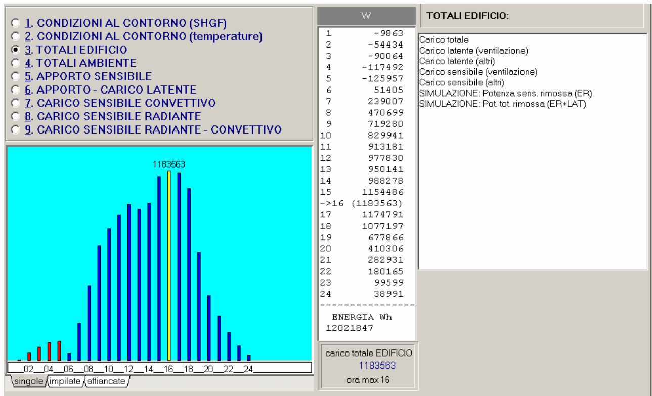
Figura 171: Carichi termici orari per il mese di giugno per l'edificio originale
