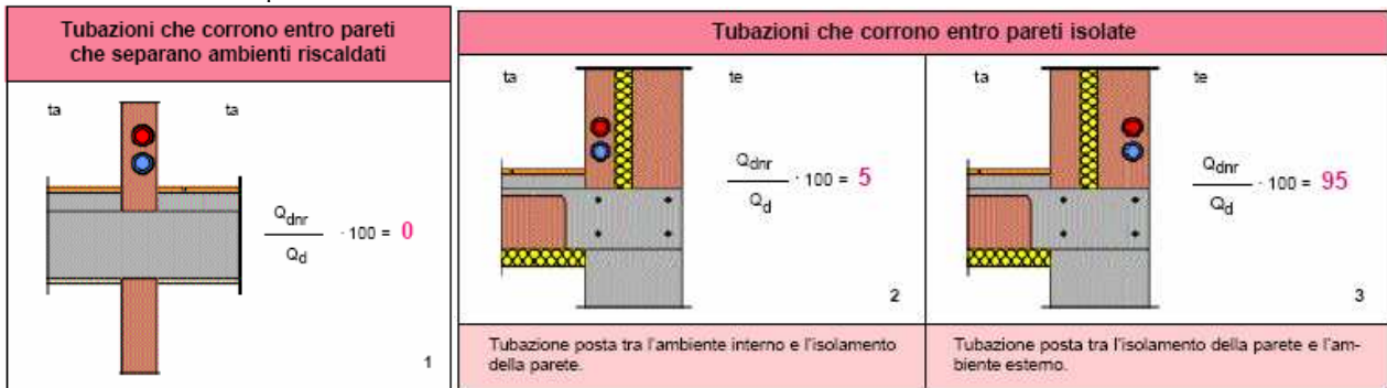
Figura 161: Effetti della posizione delle tubazioni sul rendimento di distribuzione
