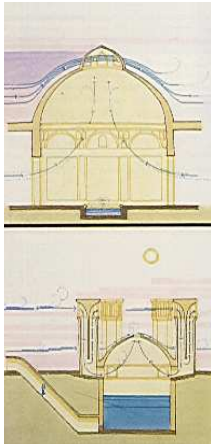
Figura 198: Schema di funzionamento delle Torri Iraniane
