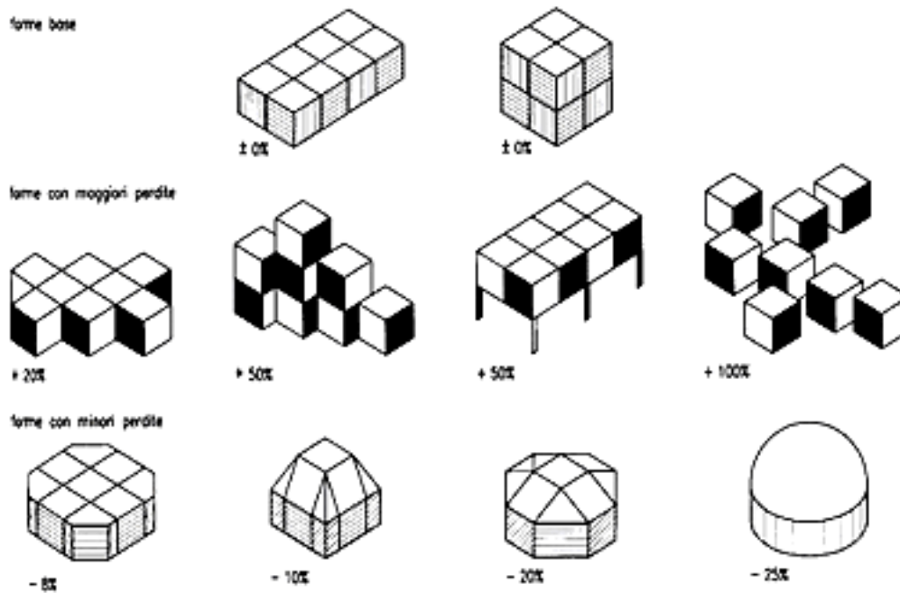
Figura 32: Influenza della forma architettonica ( A/V ) sui disperdimenti
