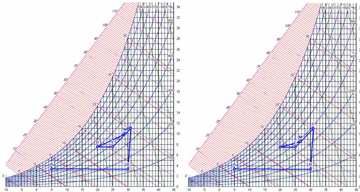
Figura 283: Regolazione invernale mediante variazione della portata del fan coil
