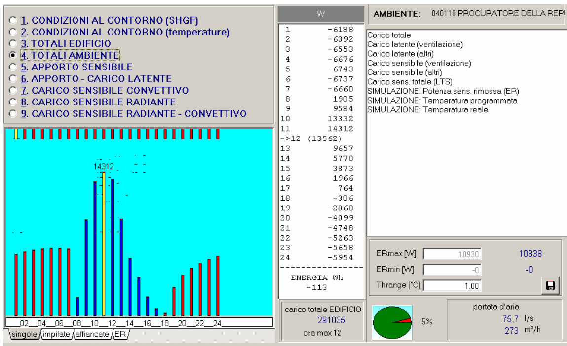
Figura 169: Carico termico a gennaio per un ambiente di riferimento a 2° piano per l'edificio originale
