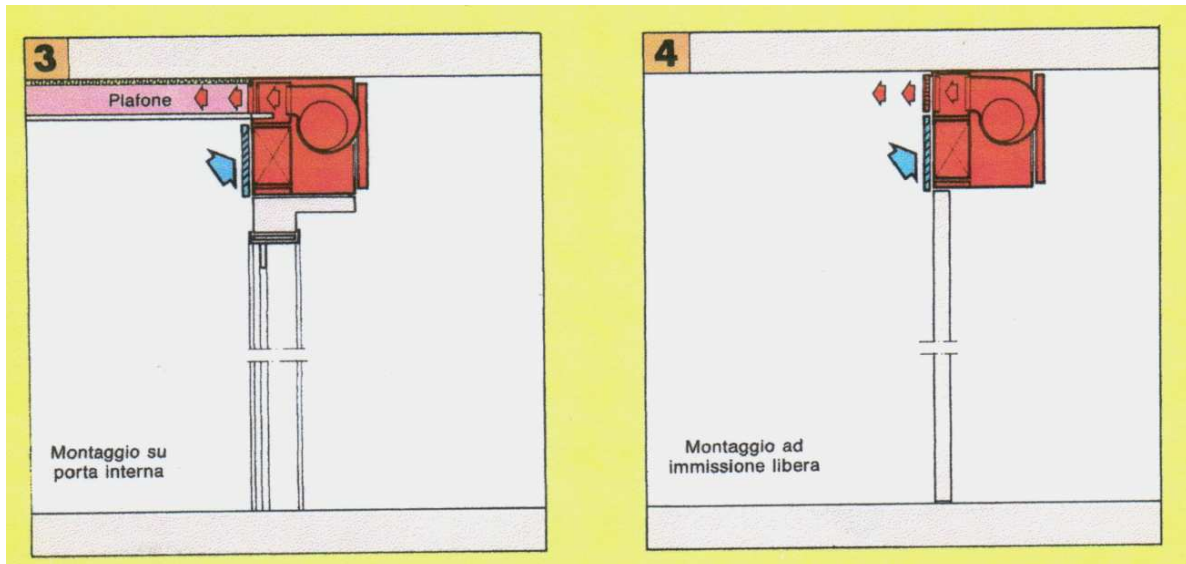
Figura 286: Disposizione dei fan coil canalizzati
