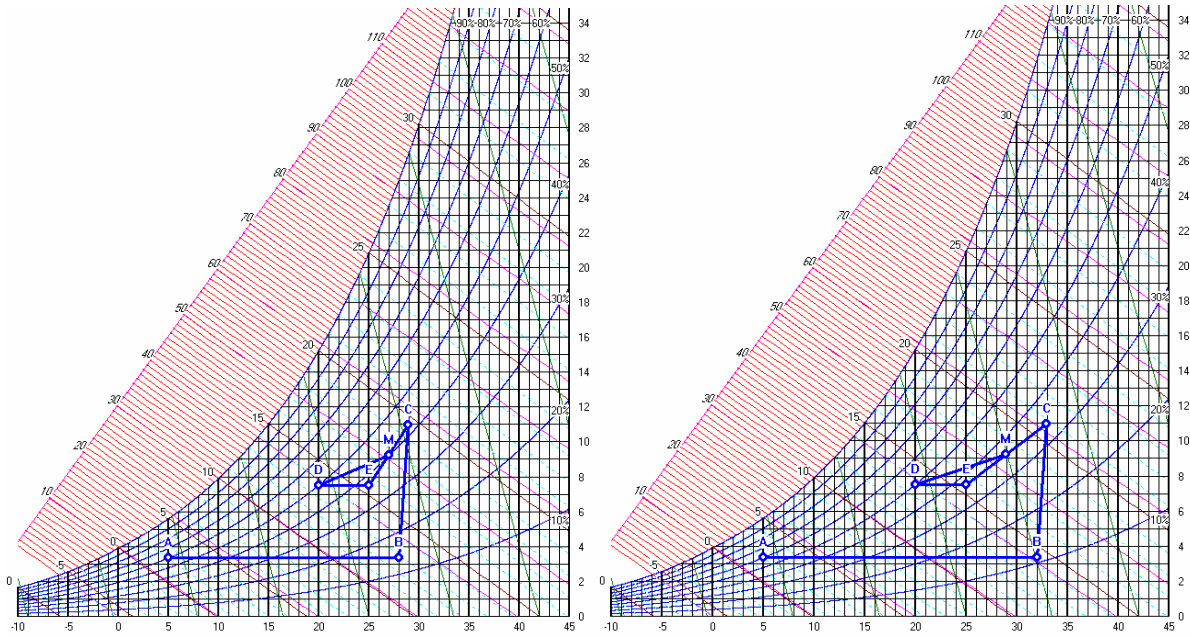
Figura 284: Regolazione invernale mediante variazione della temperatura dell'aria primaria
