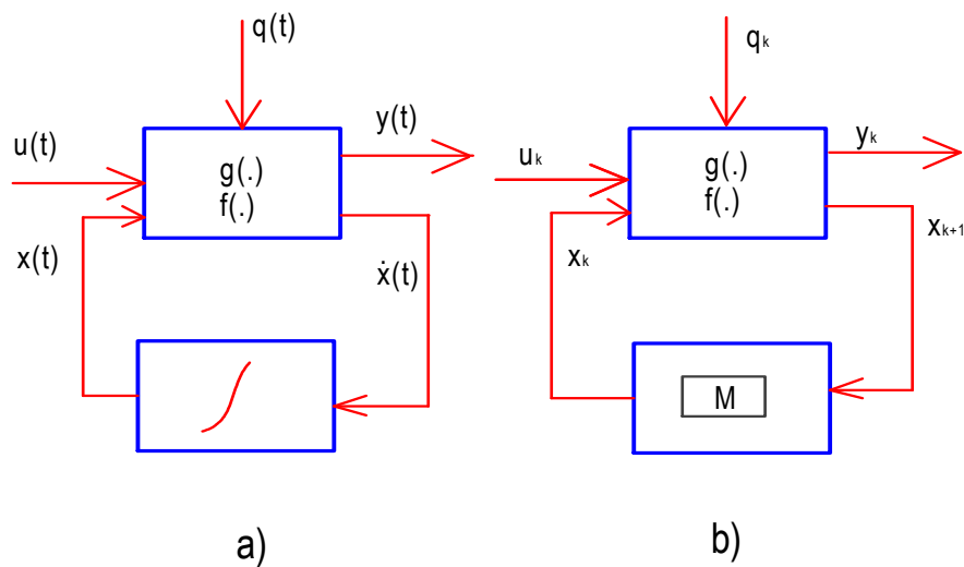
Figura 203: Rappresentazione dei sistemi dinamici continui e discreti
