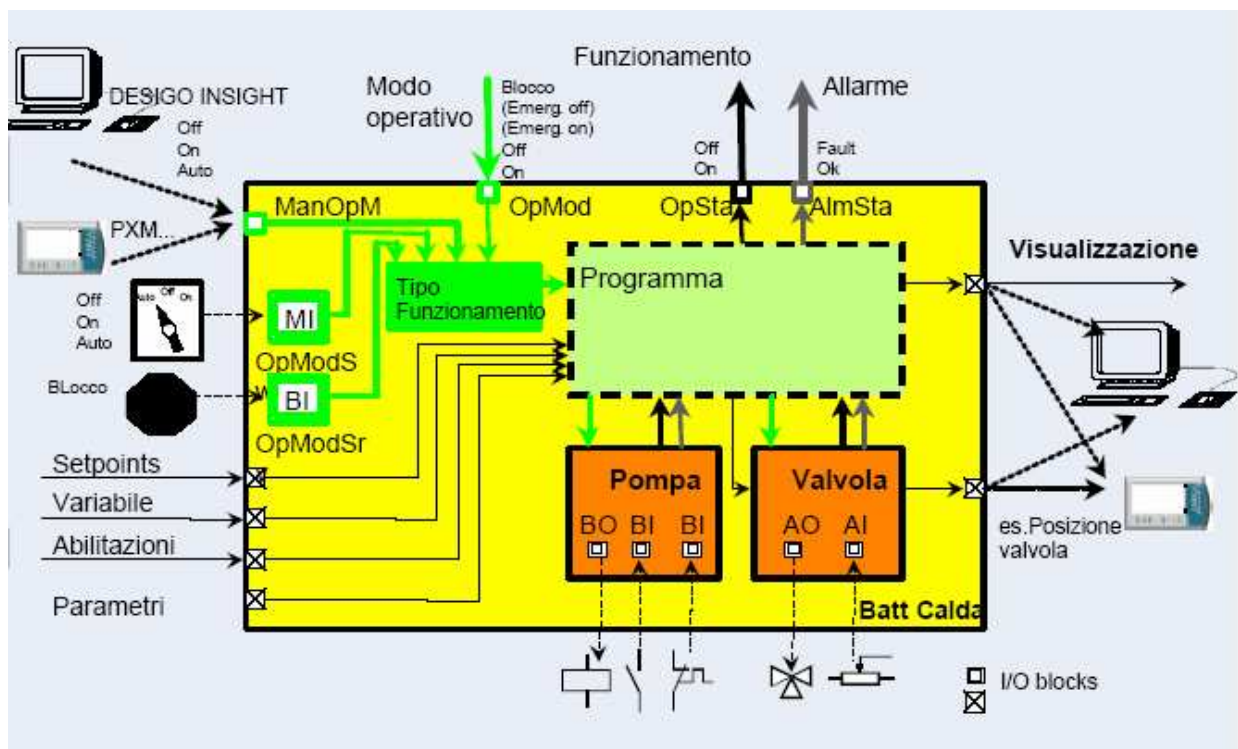
Figura 326: Configurazione dei set point di un controller
