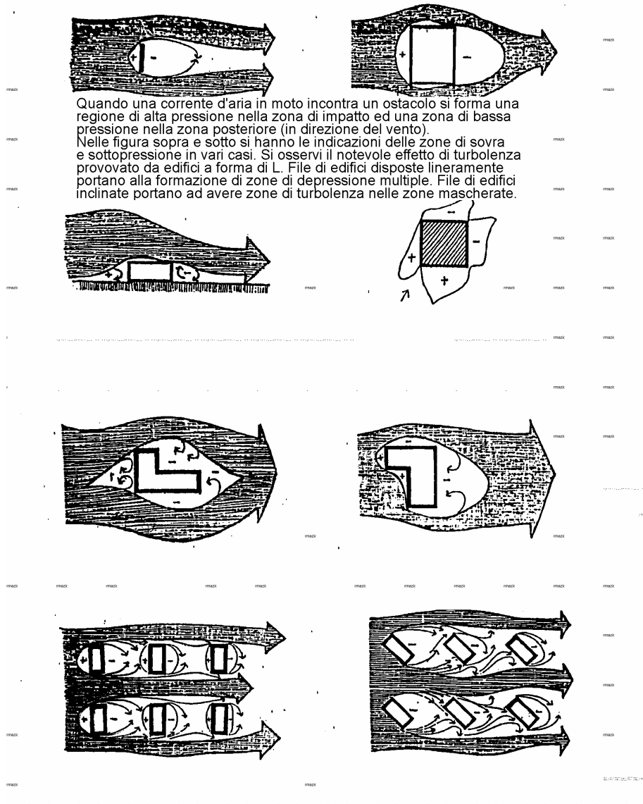
Figura 194: Zone sopra e sotto vento
