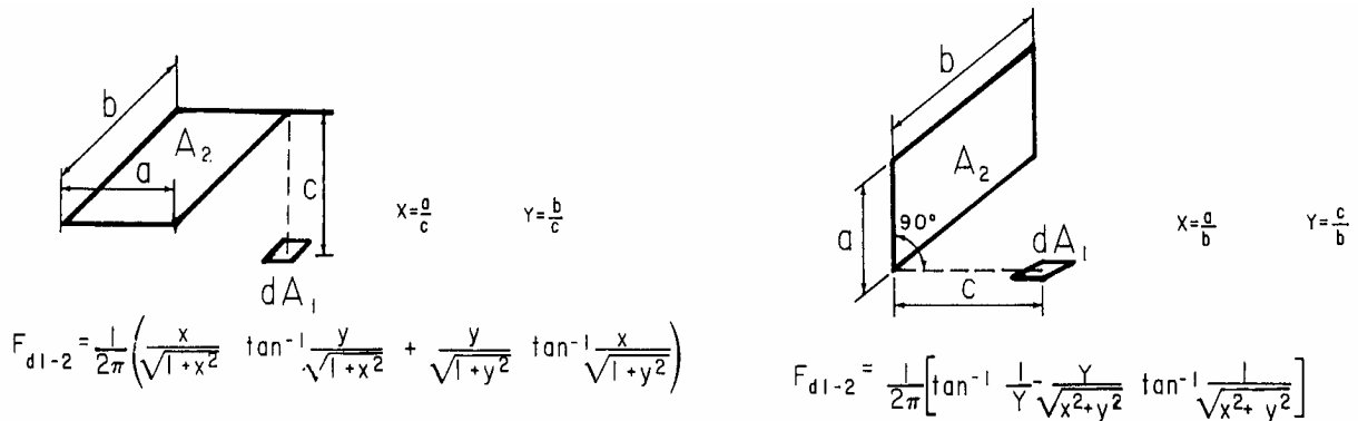
Figura 19: Formule analitiche del fattore di vista per piccoli piani
