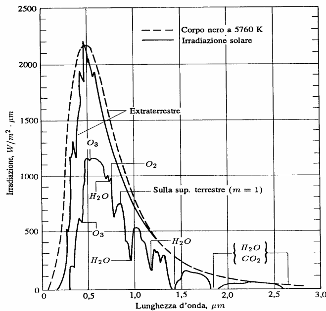
Figura 40: Radiazione solare fuori dell'atmosfera e al suolo
