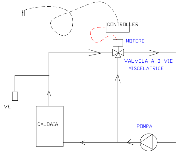
Figura 302: Sistema di regolazione con valvola a 3 vie miscelatrice
