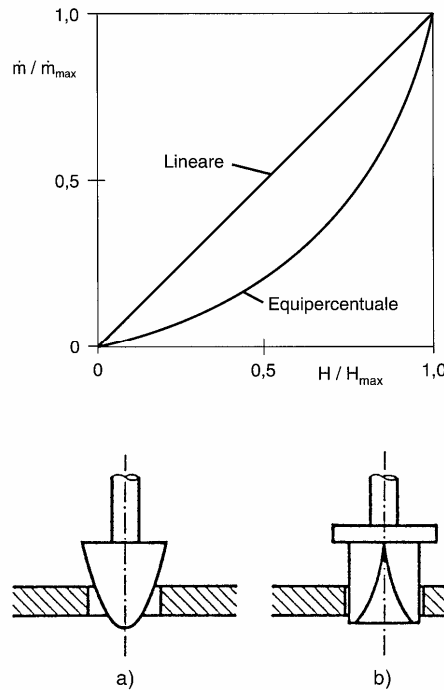
Figura 307: Curve caratteristiche lineari ed equipercentuale di una valvola
