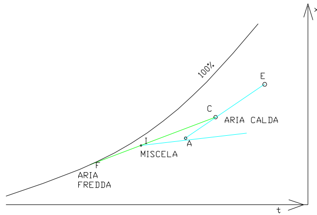
Figura 254: Miscelazione dell'aria in un impianto a doppio canale
