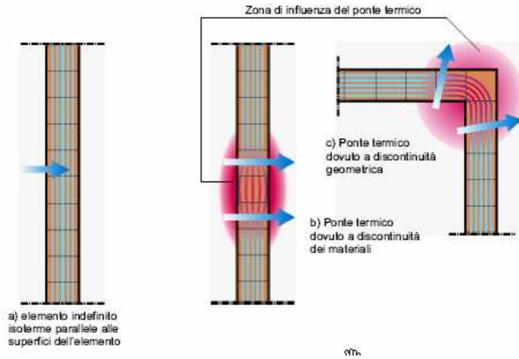
Figura 136: Trasmissione di calore attraverso i ponti termici
