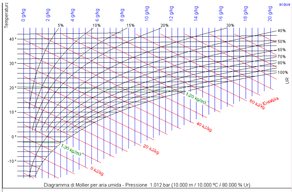
Figura 131: Diagramma di Mollier per p_t=1.012 \text{ bar}
