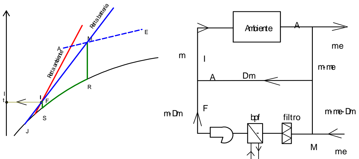
Figura 239: Postriscaldamento a miscela
