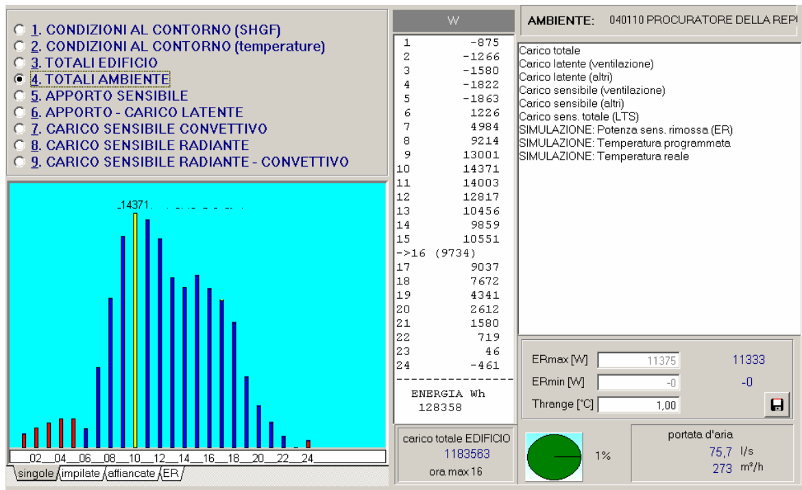
Figura 173: Carico termico orario per il 21 giugno in un ambiente di riferimento 2° piano edificio originale
