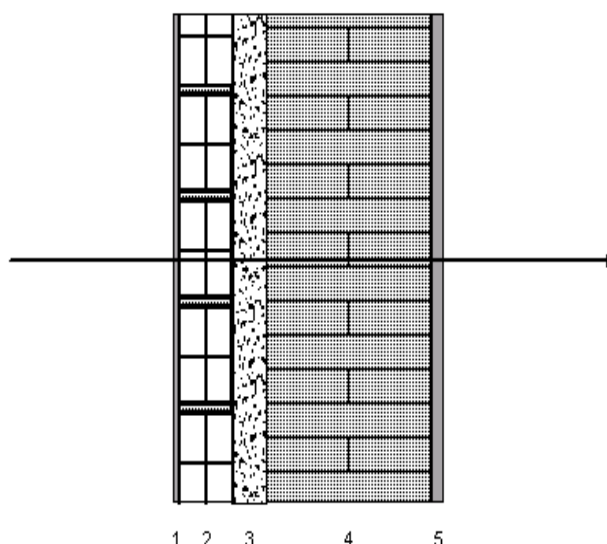
Figura 129: Stratigrafia di una parete composta
