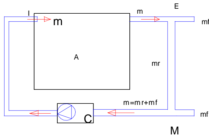
Figura 213: Schematizzazione di un impianto a tutt'aria con ricircolo
