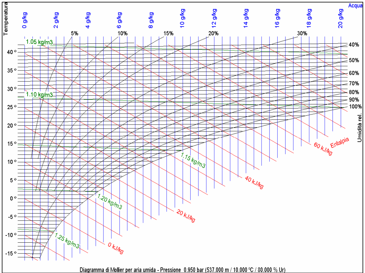
Figura 118: Diagramma psicrometrico di Mollier
