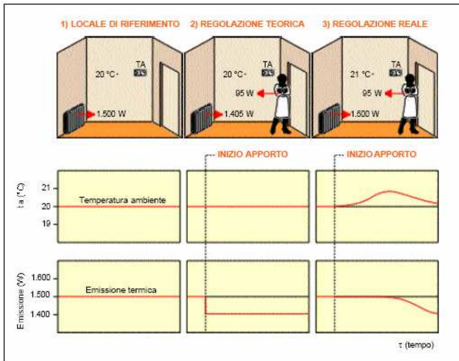
Figura 160: Schema della regolazione della temperatura ambientale
