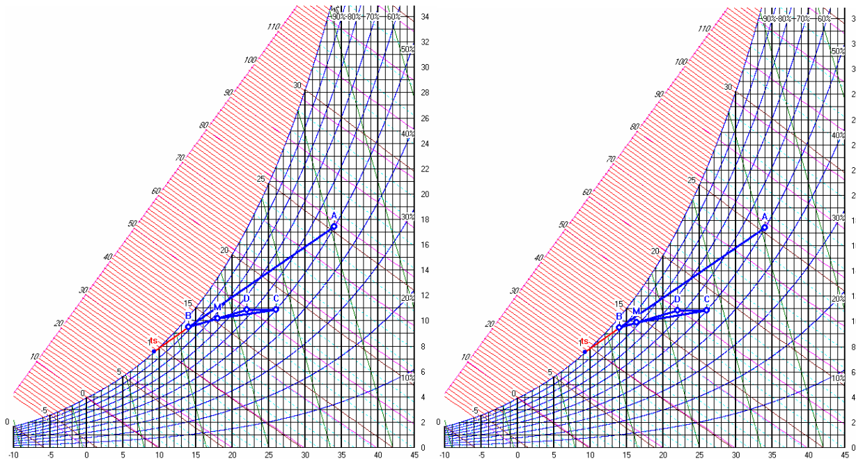
Figura 281: Regolazione estiva mediante variazione della portata di FC
