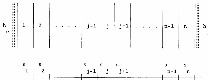
Figura 42: Schematizzazione di una parete multistrato
