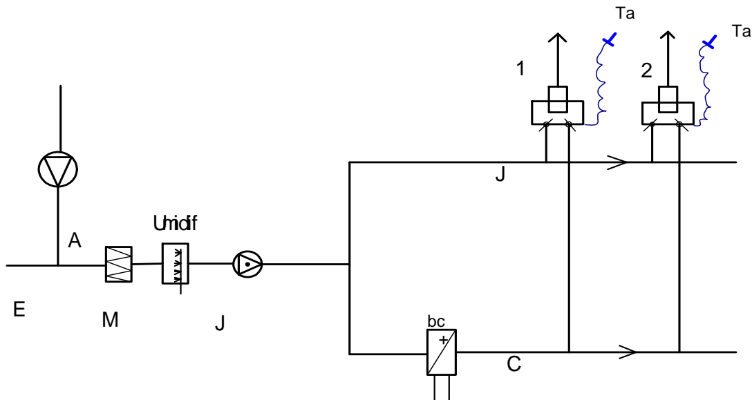
Figura 260: Schema impianto dual conduit in regime invernale
