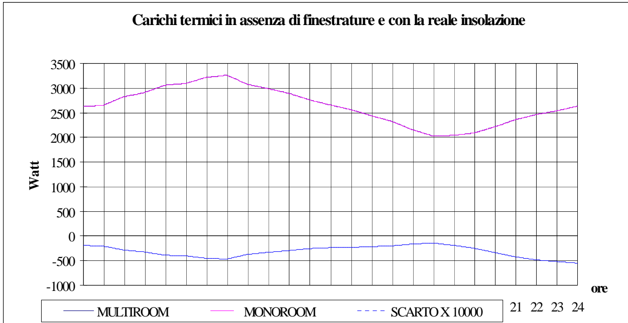
Figura 53: Andamento dei carichi termici senza finestre
