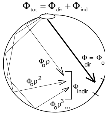
Figura 45: Schematizzazione degli scambi radiativi
