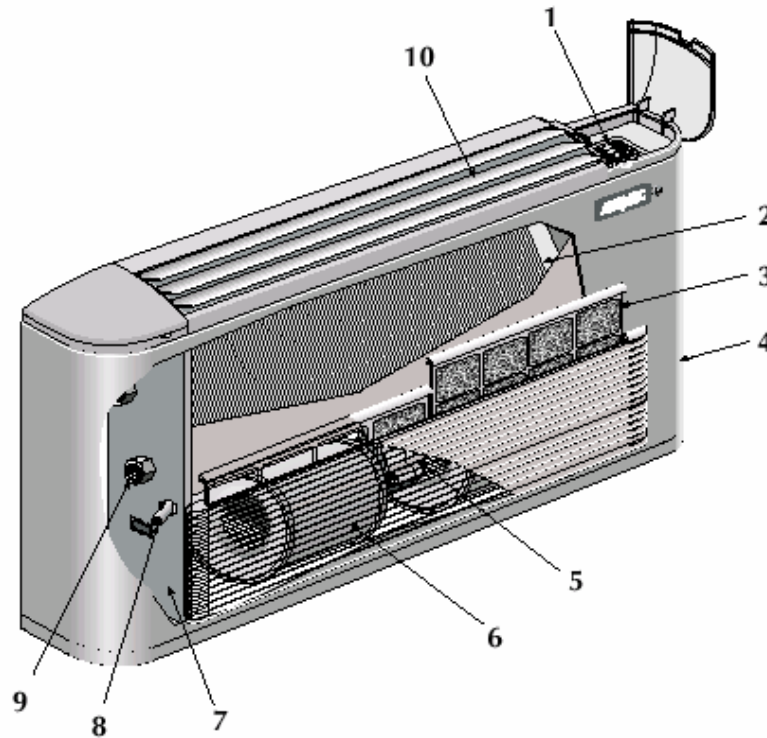
Figura 270: Sezione con particolari costruttivi di un moderno fan coil
