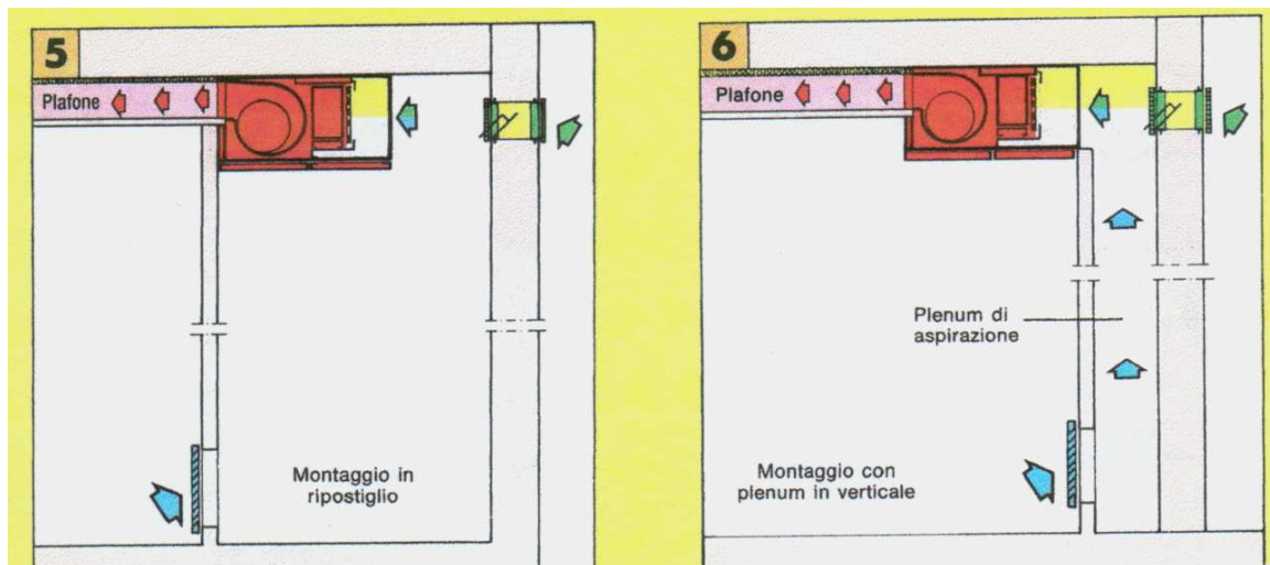
Figura 290: Disposizione dei fan coil canalizzati
