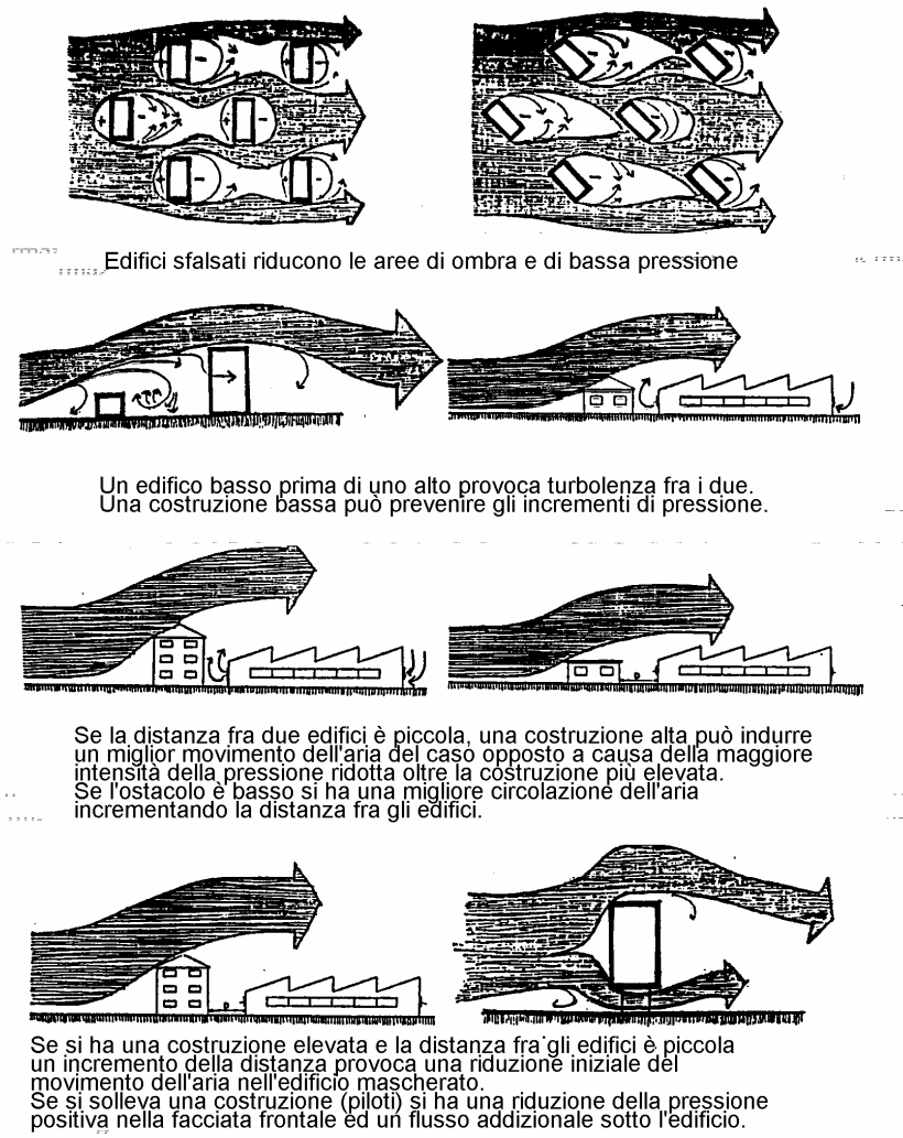
Figura 193: Effetti del vento e modificazioni apportate dagli edifici
