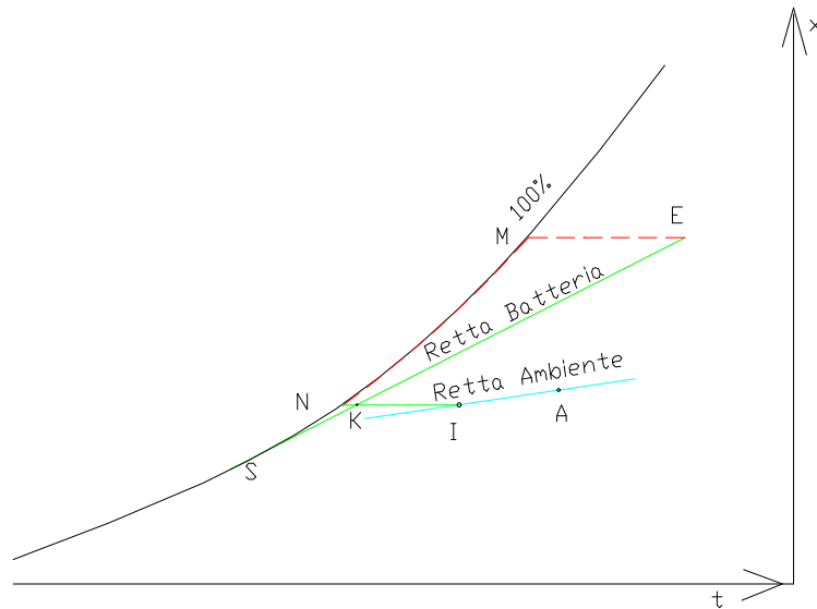
Figura 241: Ciclo estivo senza ricircolo con postriscaldamento – ASHRAE
