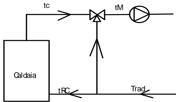
Figura 334: Caldaia con valvola a tre vie
