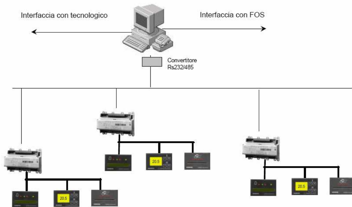
Figura 330: Insieme di controller locali collegati in rete ad una unità centrale
