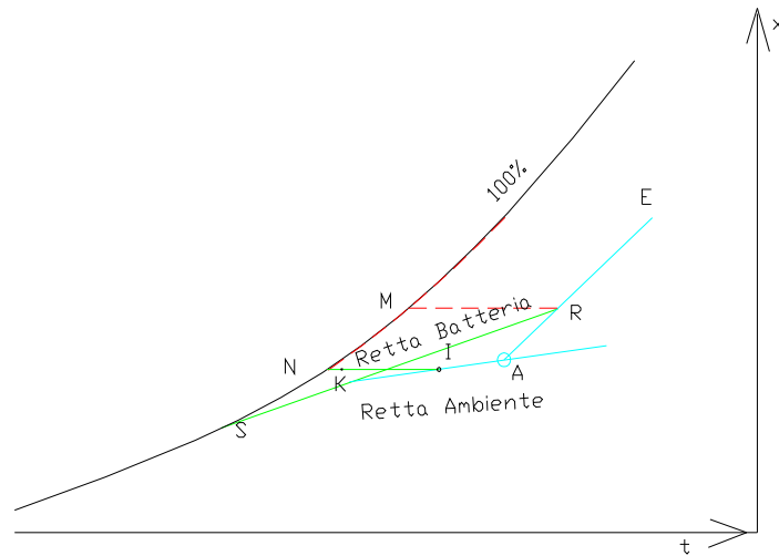
Figura 245: Ciclo estivo con ricircolo e postriscaldamento – ASHRAE
