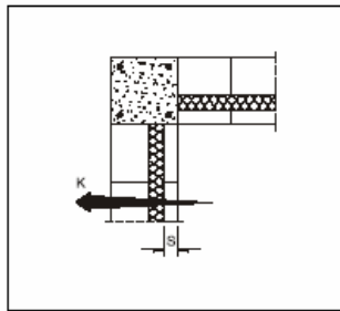
Figura 136: Trasmissione di calore attraverso i ponti termici
