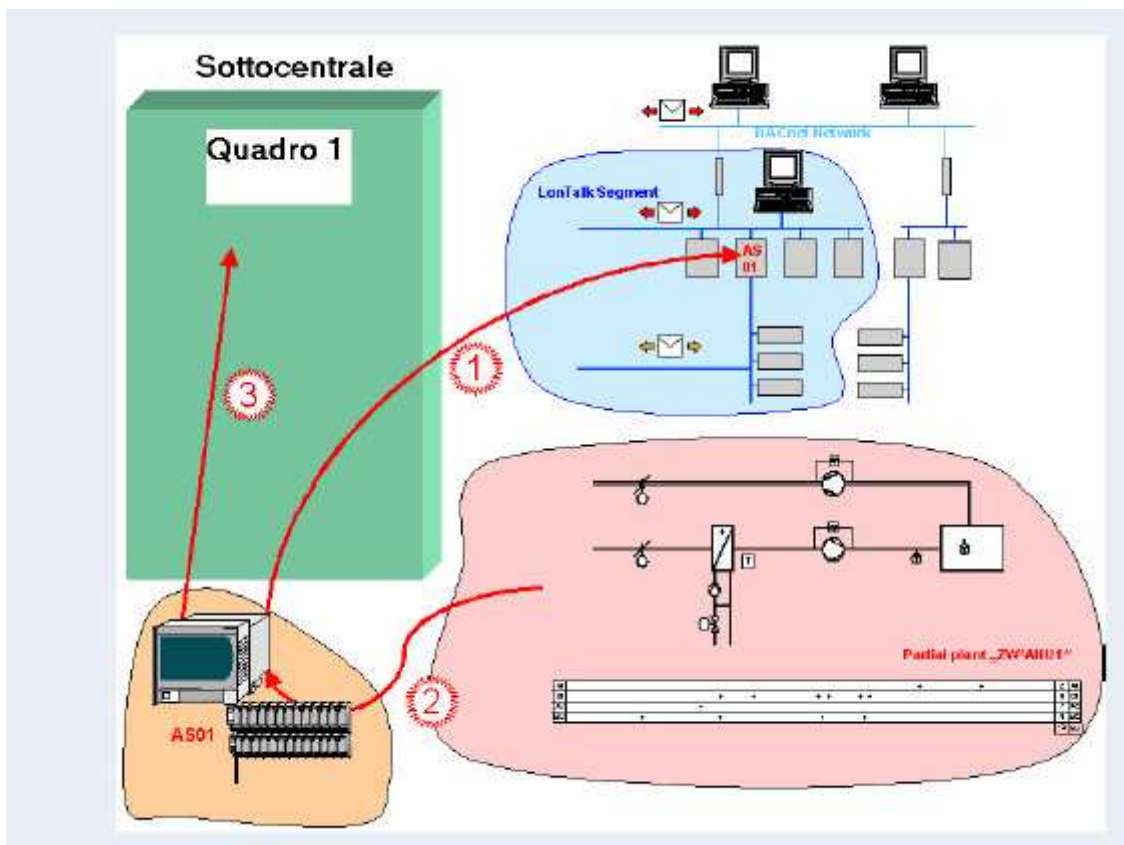
Figura 329: Schema di collegamento delle apparecchiature al bus
