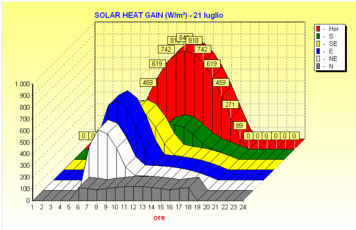
Figura 172: Andamento della radiazione solare per il giorno 21 luglio a Modica
