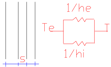
Figura 36: Schematizzazione di una parete con intercapedine
