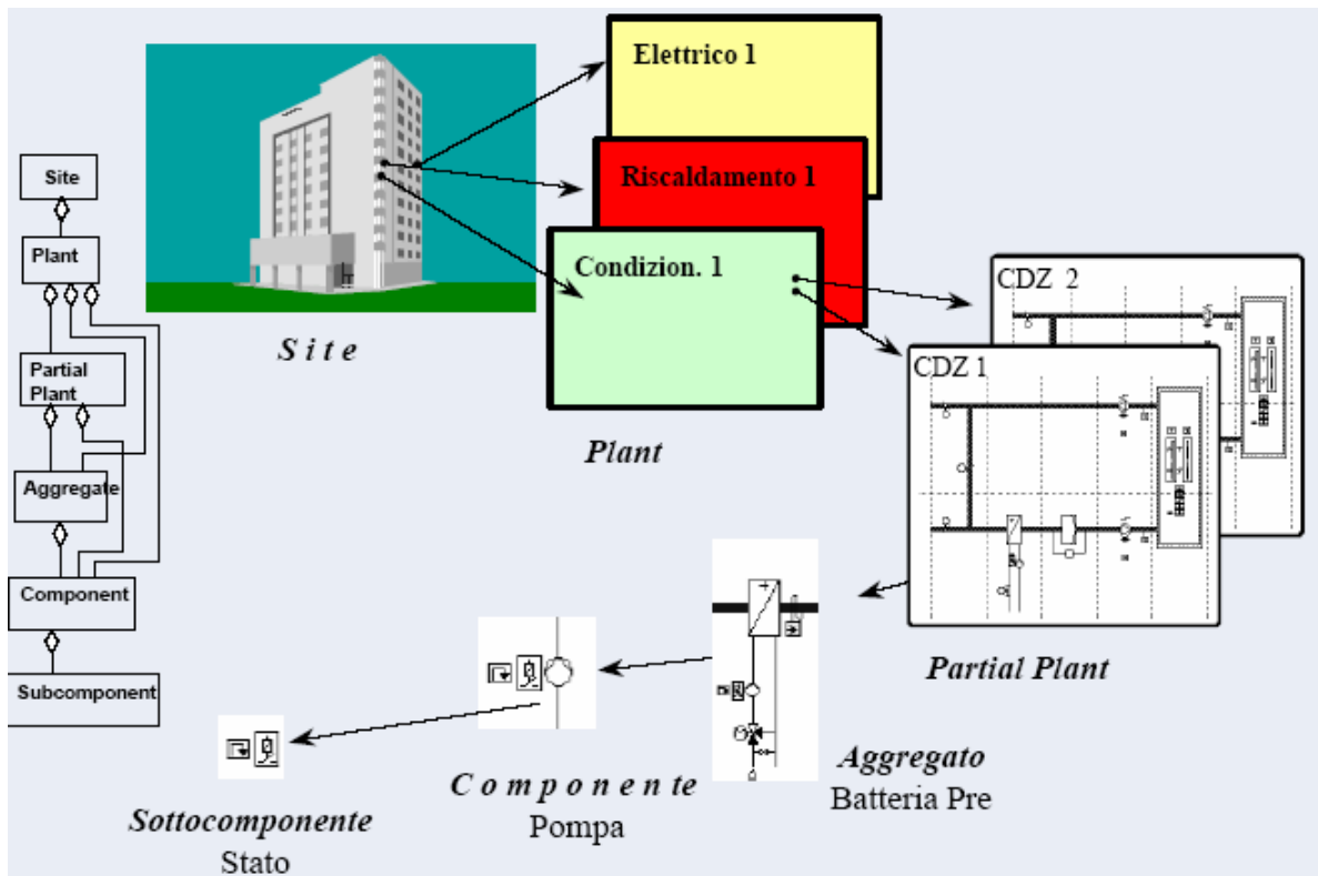
Figura 317: Gestione integrata di tutti gli impianti di un edificio
