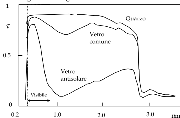
Figura 165: Finestra di trasparenza del vetro
