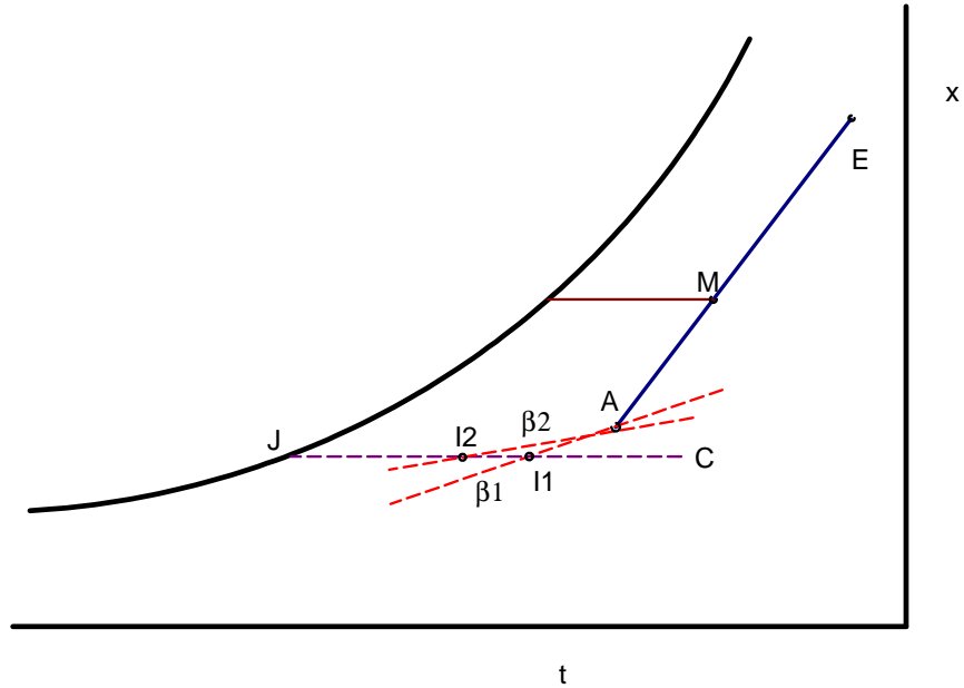
Figura 259: Trasformazioni per dual conduit in regime estivo per schema alternativo
