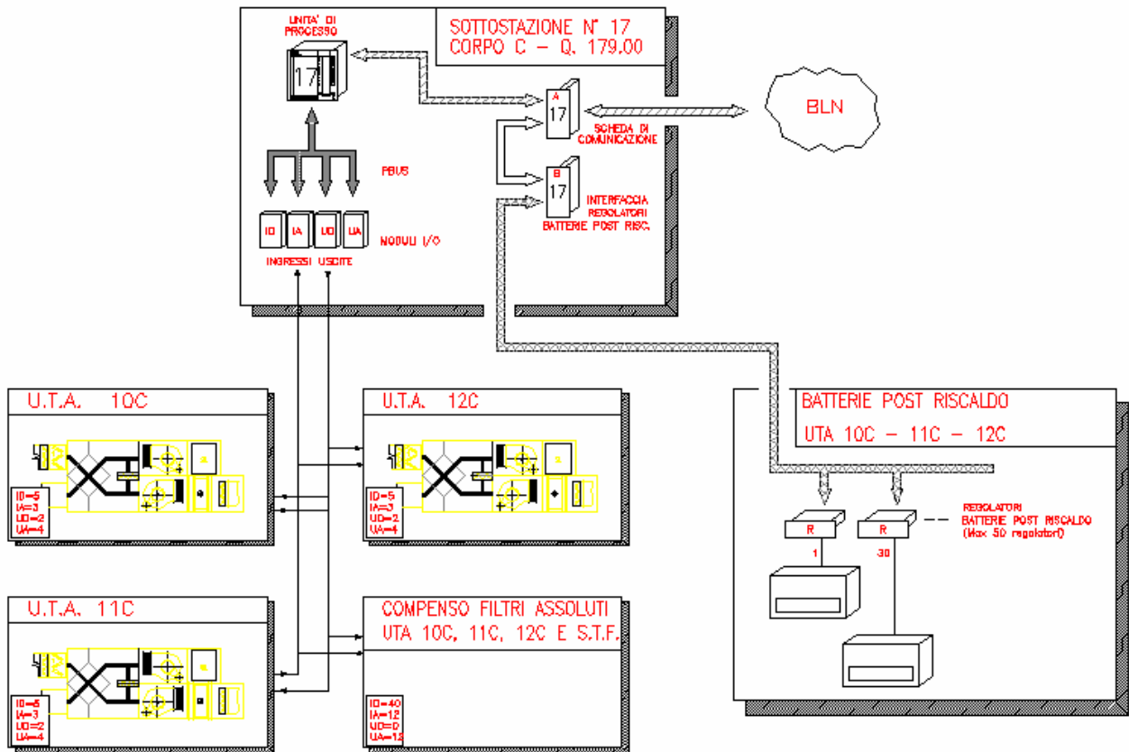
Figura 322: Esempio di collegamenti di controller locali su più dispositivi
