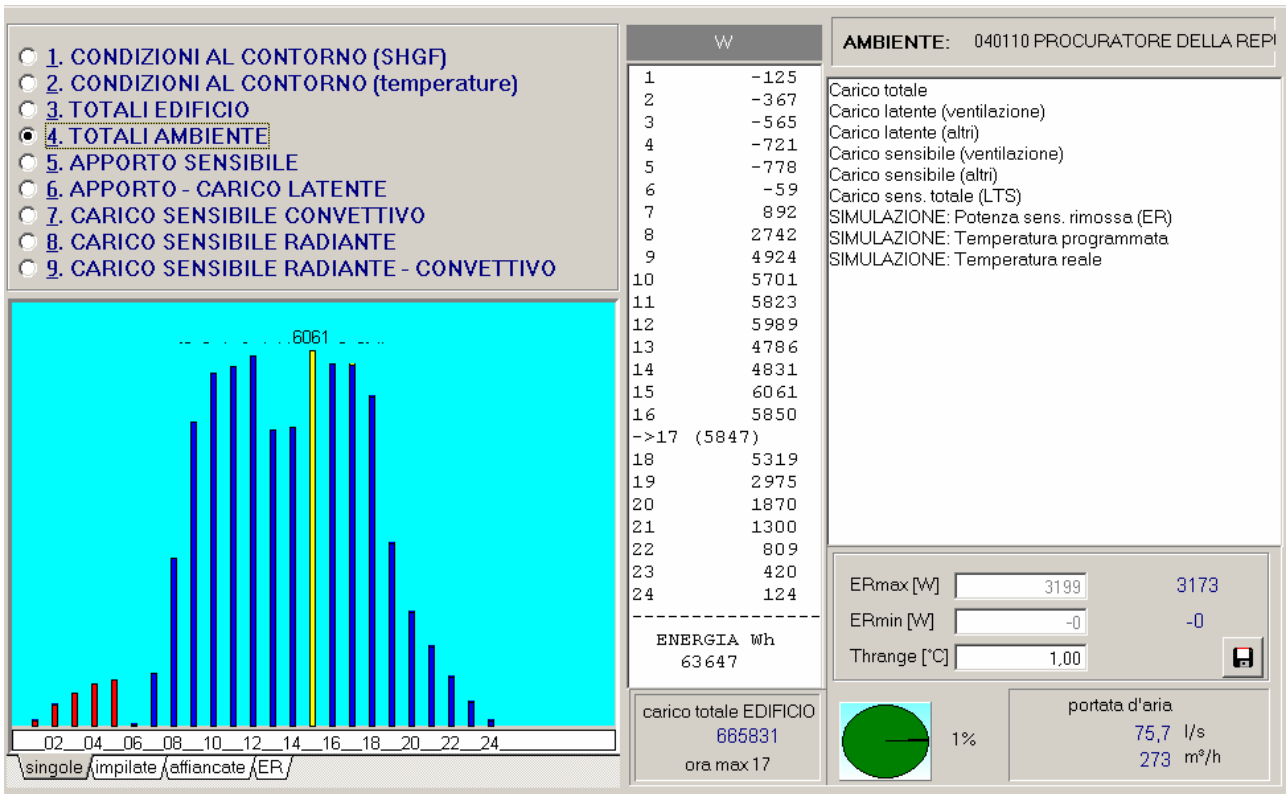
Figura 179: Carichi orari in giugno in un ambiente di riferimento al 2° piano con edificio protetto con film
