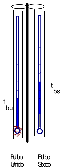
Figura 126: Psicrometro a ventolina
