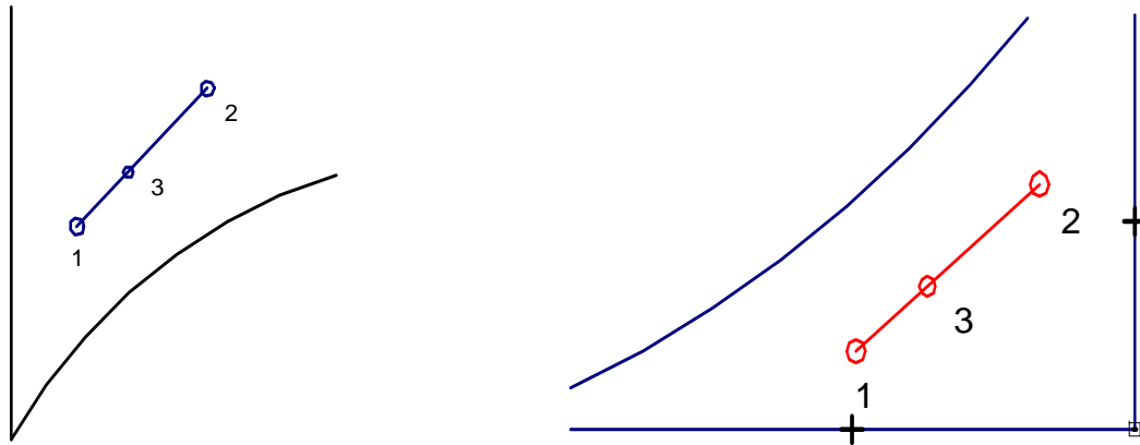
Figura 120: Rappresentazione della miscelazione adiabatica di due correnti d'aria umida
