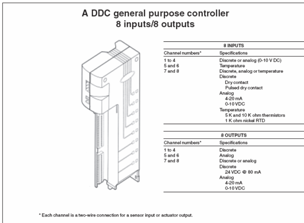
Figura 319: Esempio di controller locale con convertitori A/D e D/A incorporati
