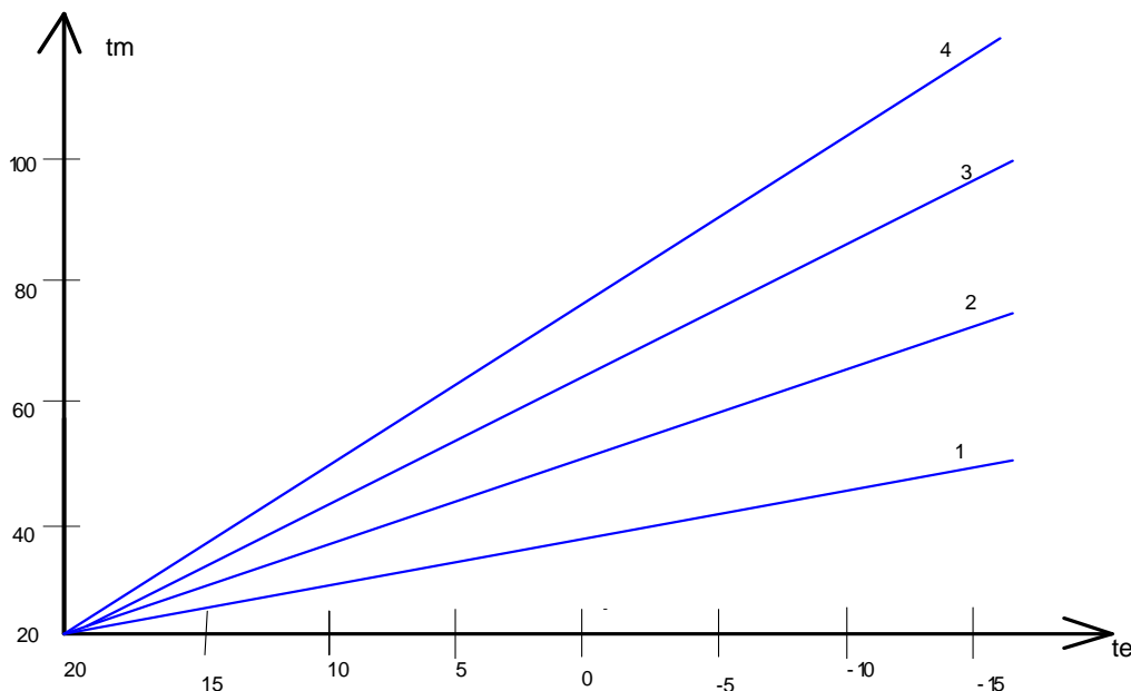
Figura 332: Curve di regolazione linearizzate
