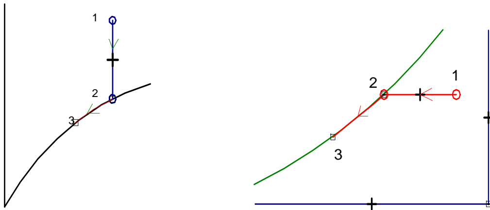
Figura 122: Rappresentazione del raffreddamento di un flusso di aria umida
