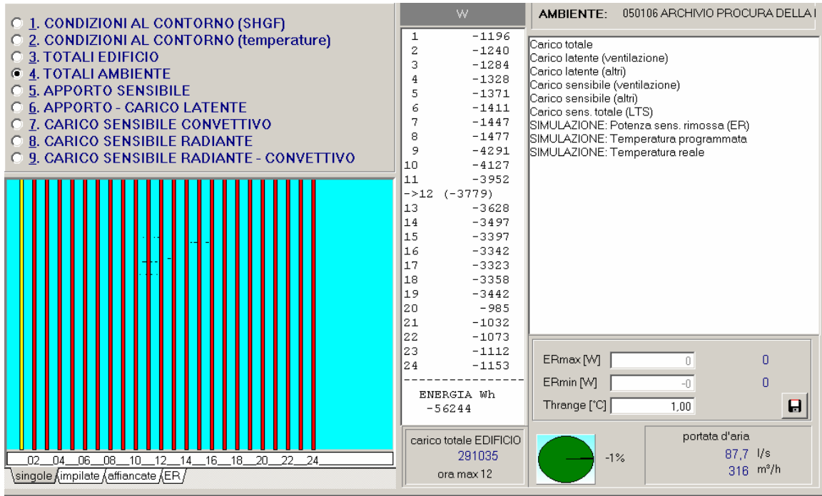
Figura 170: Carico termico a gennaio per una seconda stanza a NW a 2° piano per l'edificio originale
