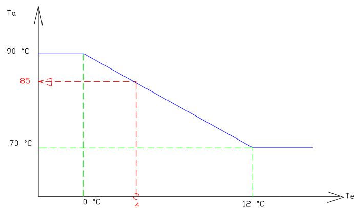
Figura 301: Regolazione della temperatura dell’acqua calda in caldaia
