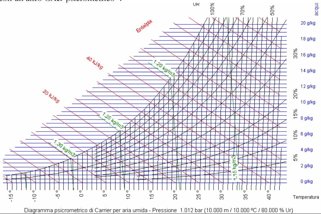
Figura 132: Diagramma ASHRAE- Carrier per p_i=1.012 bar
