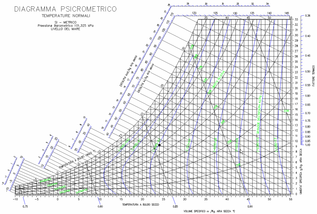
Figura 119: Diagramma psicrometrico ASHRAE
