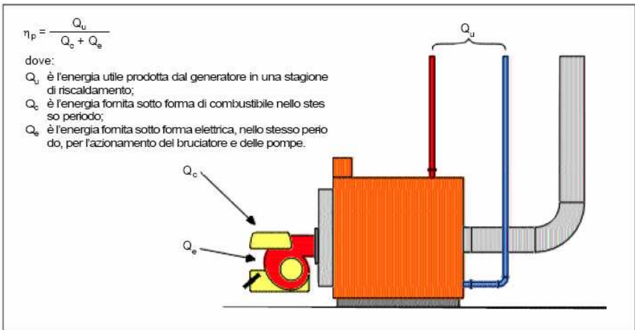
Figura 162: Rendimento di produzione
