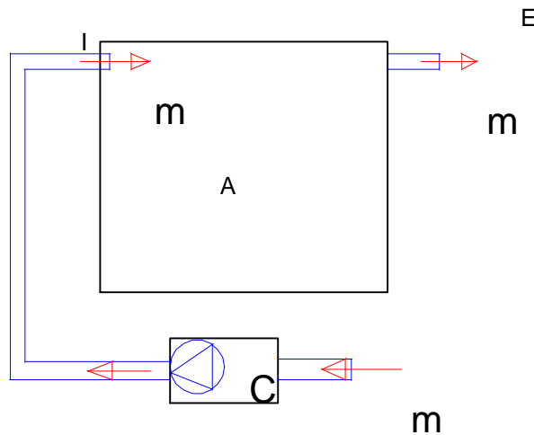
Figura 201: Schematizzazione di un impianto a tutt'aria senza ricircolo
