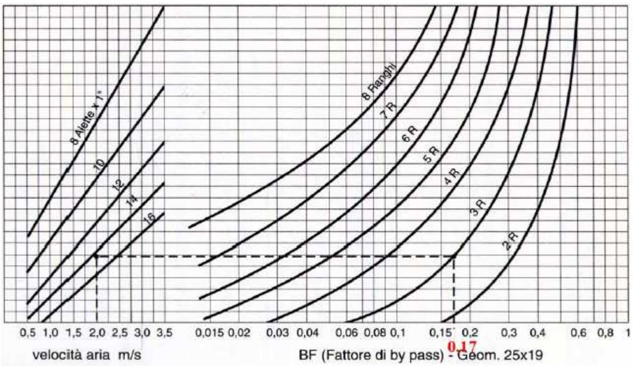
Figura 230: Calcolo del fattore di by pass per una batteria
