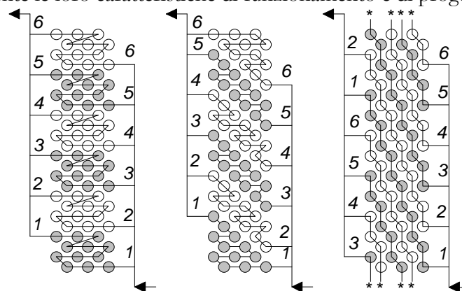
Figura 217: Tipologie di flusso nelle batterie alettate
