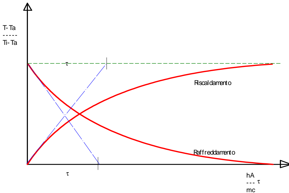
Figura 30: Andamento del transitorio di riscaldamento e/o di raffreddamento
