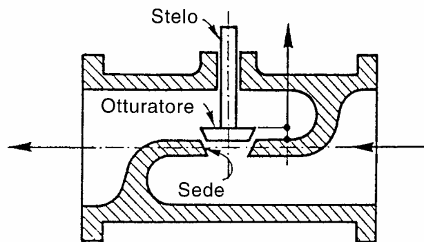
Figura 306: Schema costruttiva di una valvola
