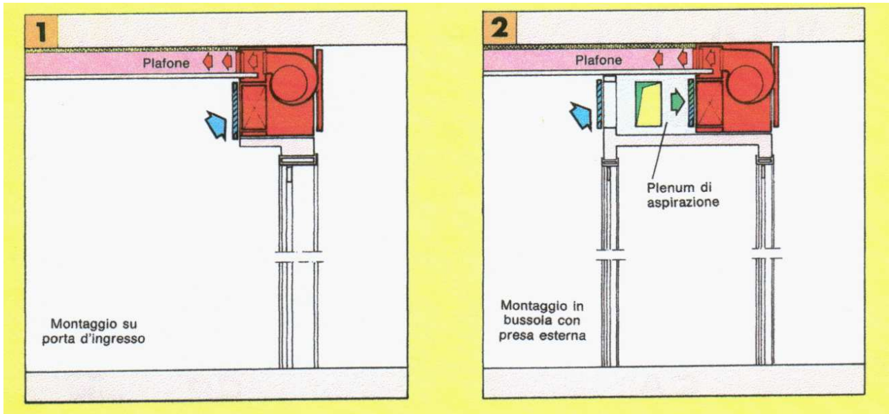
Figura 285: Disposizione dei fan coil canalizzati
