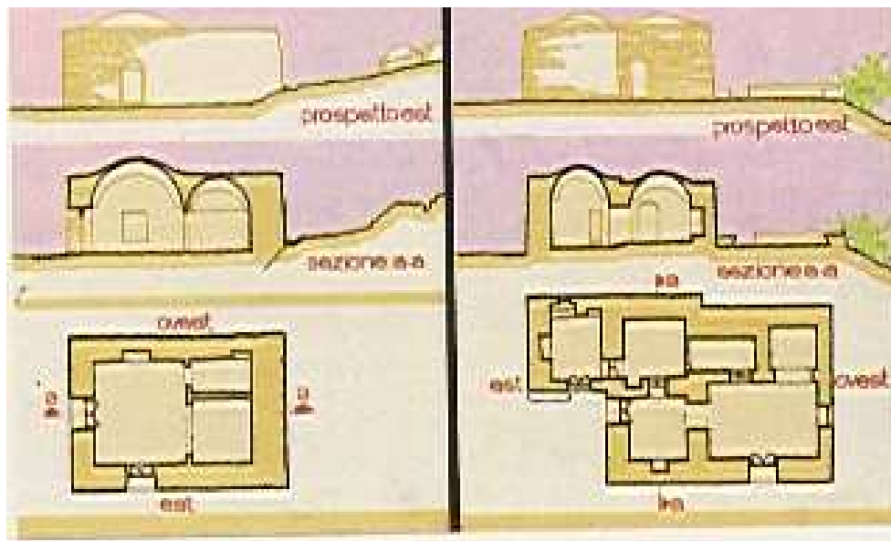
Figura 192: Schema di funzionamento di un Dammuso di Pantelleria
