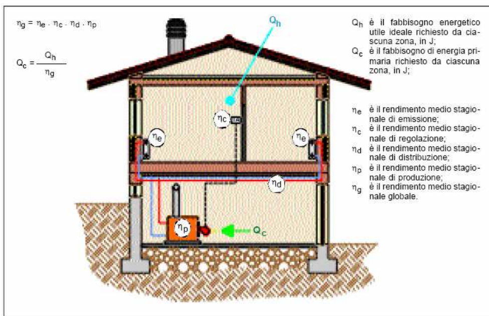
Figura 153: Schematizzazione dell'interazione edificio-impianto
