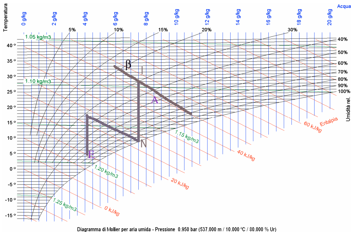
Figura 212: Trasformazioni ideali per condizionamento invernale senza ricircolo
