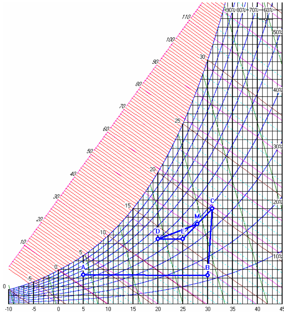
Figura 278: Schema di funzionamento di un impianto AP + FC invernale
