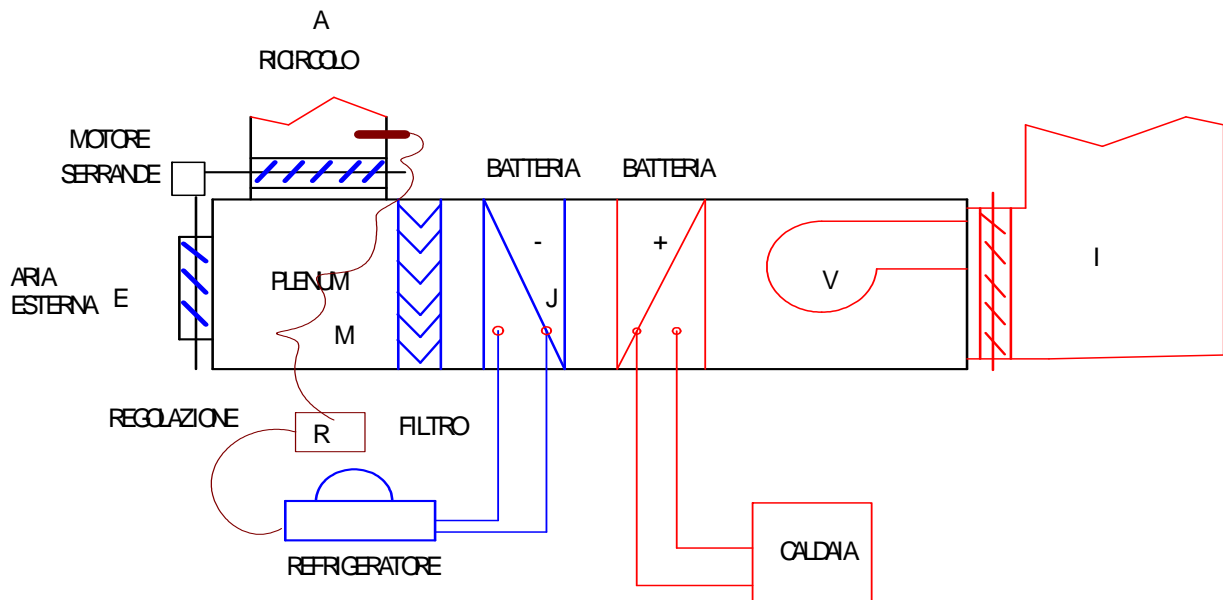
Figura 343: Regolazione on-off di una batteria ad espansione diretta
