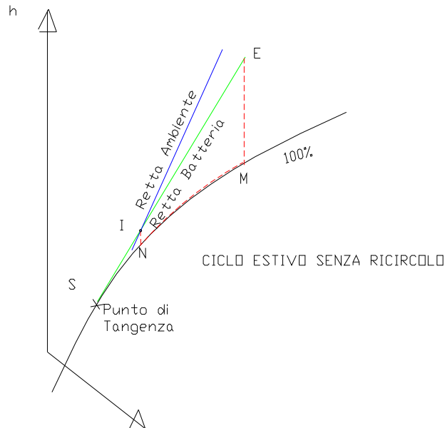
Figura 232: Rappresentazione del ciclo estivo senza ricircolo
