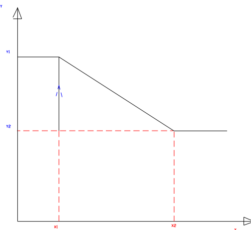
Figura 305: Funzione di risposta di un regolatore ad azione proporzionale
