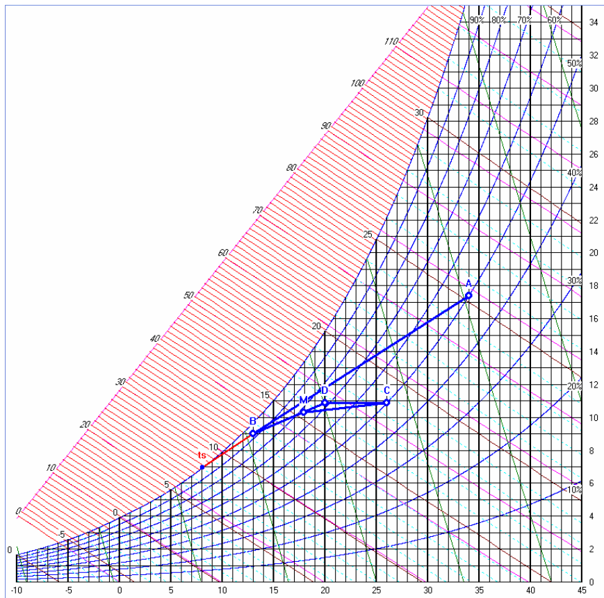
Figura 275: Rappresentazione di un impianto misto nel piano psicrometrico
