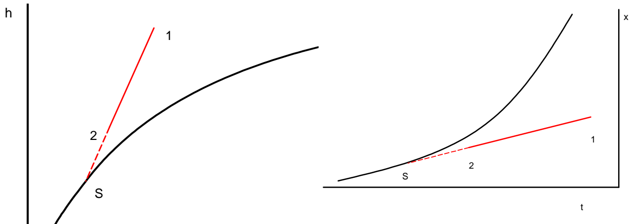
Figura 227: Deumidificazione nel piano di Mollier ed ASHRAE
