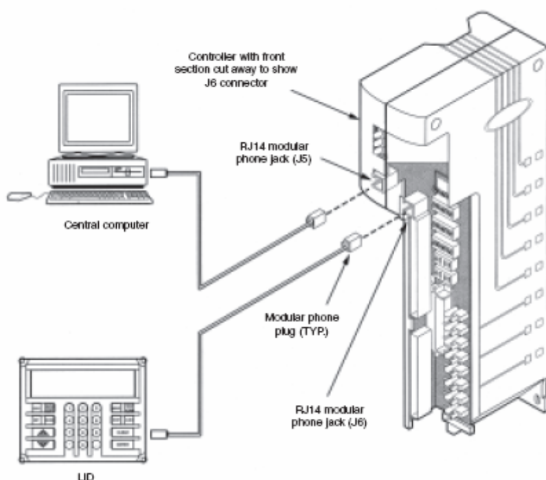
Figura 327: Collegamento del controller locale al supervisor e all'unità di programmazione
