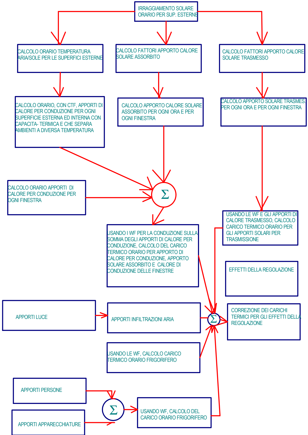
Figura 206: Schema a blocchi del Metodo TFM
