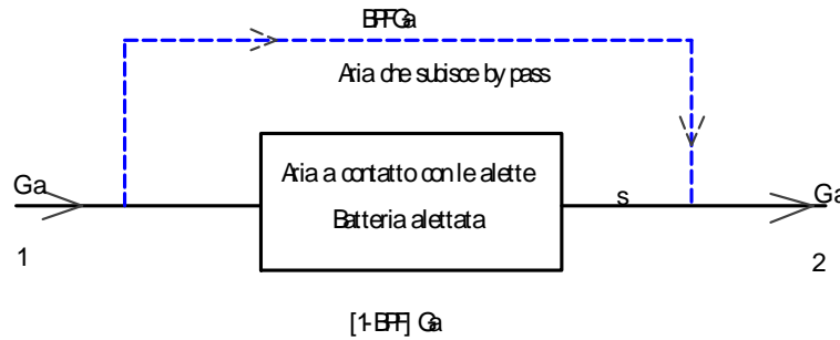
Figura 228: Schema ideale del raffreddamento con deumidificazione
