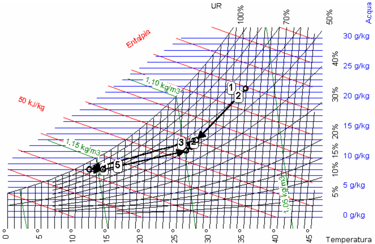
Figura 249: Ciclo estivo con ricircolo e postriscaldamento nel piano ASHRAE
