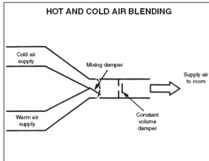
Figura 356: Miscelatore di aria per sistemi a doppio condotto
