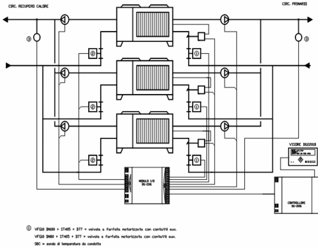
Figura 311: Esempio di regolazione computerizzata di 3 refrigeratori d'acqua
