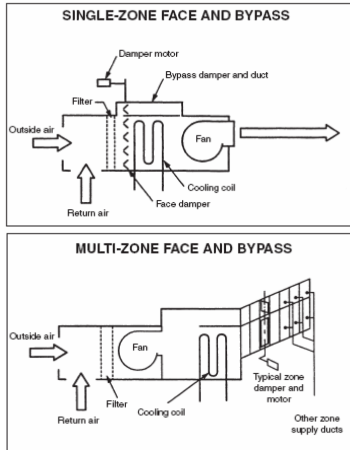
Figura 354: Controllo mediante by pass per singola zona e multizona
