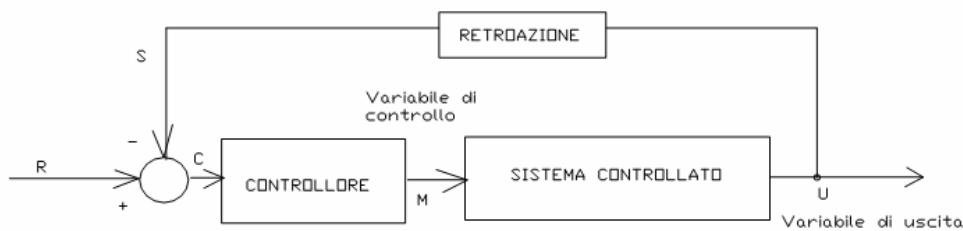
Figura 300: Sistema di regolazione a controreazione, Circuito chiuso
