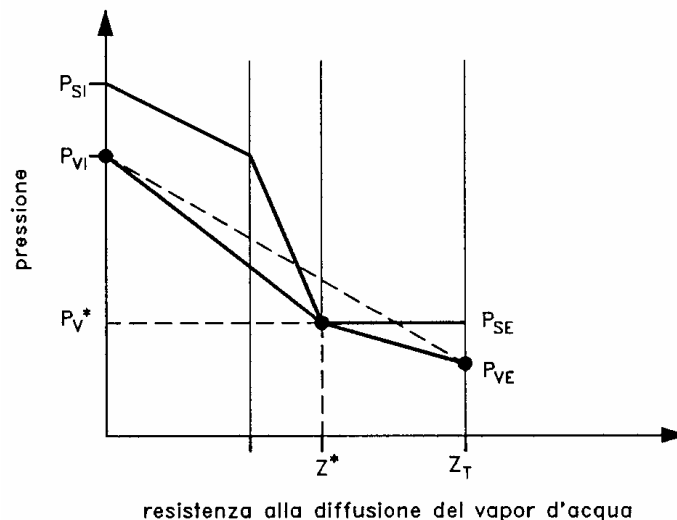
Figura 128: Diagramma di Glaser per il caso di formazione di condensa
