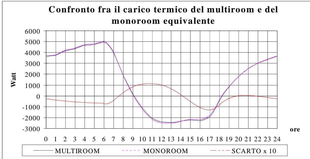
Figura 51: Andamento del carico termici per modelli multi e mono room equivalente
