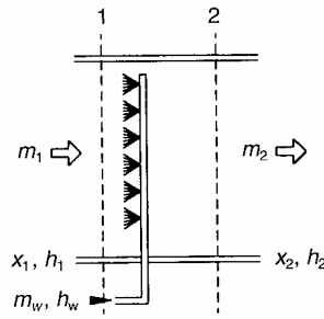
Figura 124: Schematizzazione del saturatore adiabatico ad acqua fredda
