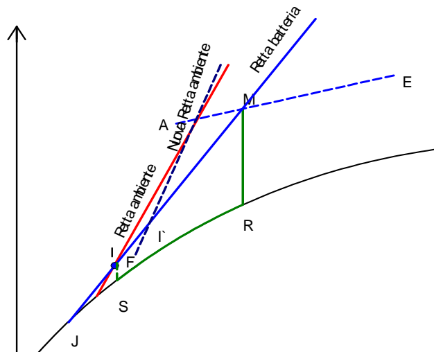
Figura 344: Regolazione del carico sensibile per un ambiente
