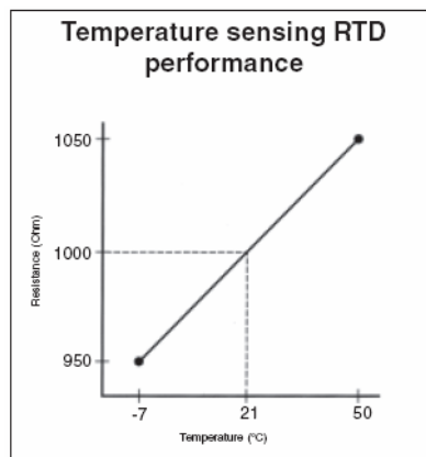
Figura 318: Linearità di un sensore di temperatura
