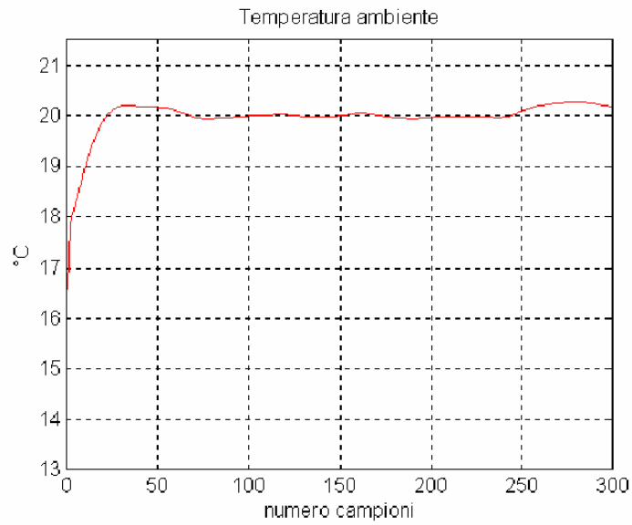
Figura 295: Andamento della temperatura interna prevista dal controller neurale
