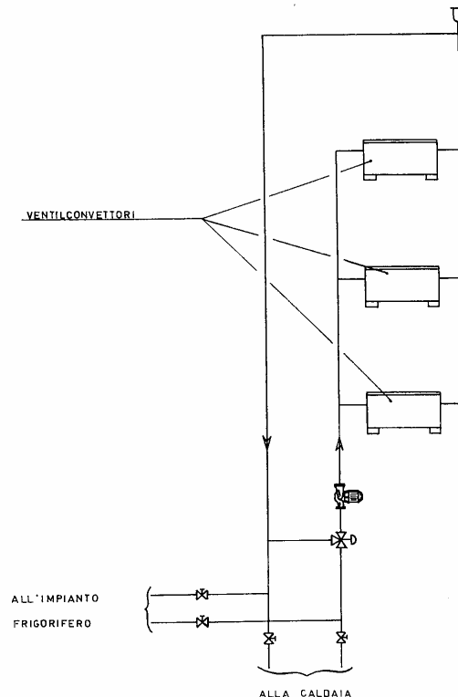
Figura 264: Rete di distribuzione dell'acqua fredda del tipo bitubo
