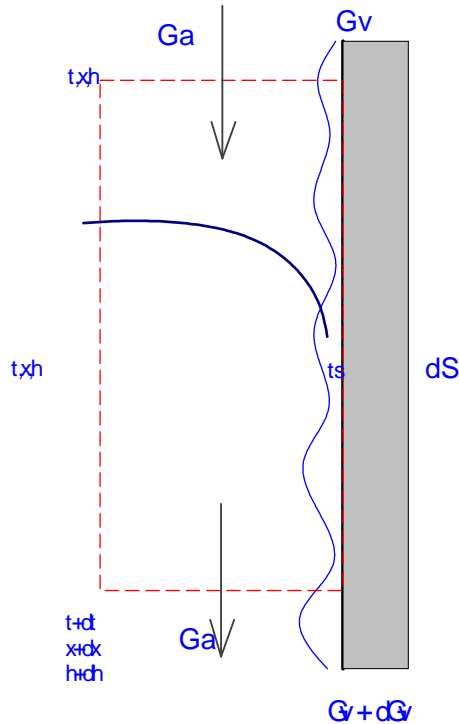
Figura 226: Bilancio di massa per il processo di deumidificazione
