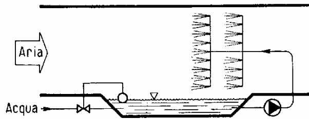
Figura 223: Schema impiantistico di un umidificatore adiabatico con spruzzi d'acqua
