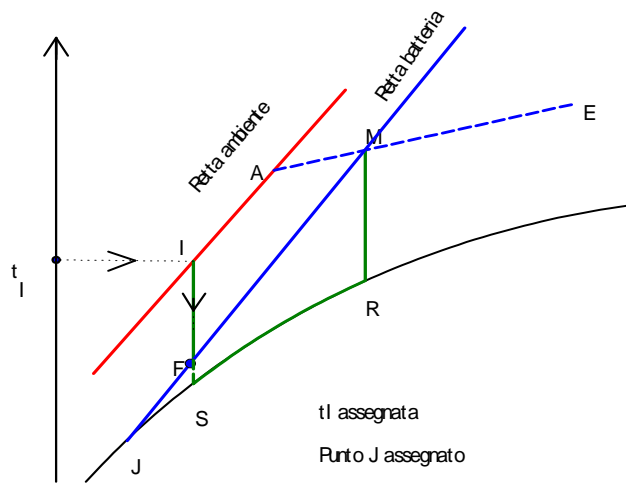
Figura 236: Retta ambiente non interseca la curva di saturazione: caso B
