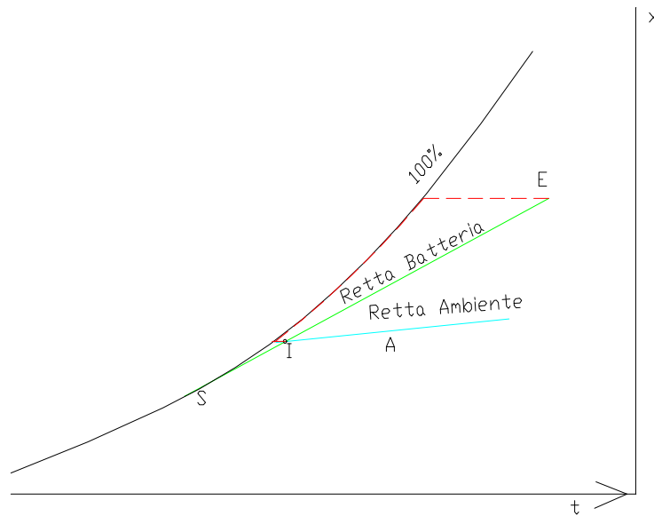
Figura 240: Ciclo estivo senza ricircolo – ASHRAE
