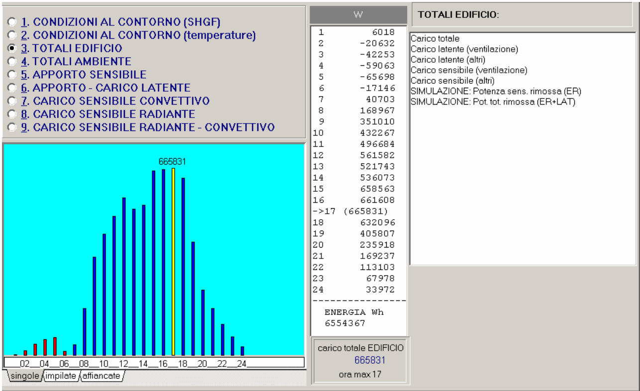
Figura 178: Carichi termici orari per il mese di giugno per l'edificio protetto con film riflettente
