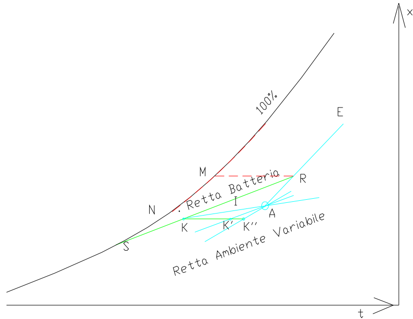
Figura 252: Variazione del punto di immissione al variare della retta ambiente
