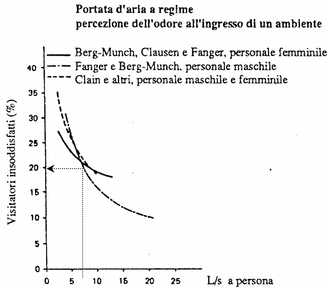
Figura 22: Relazione fra PPD e portata di aria di ventilazione
