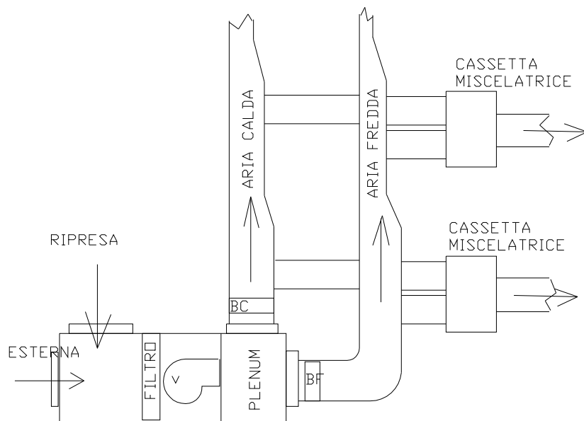
Figura 253: Schema di un impianto Dual Conduit
