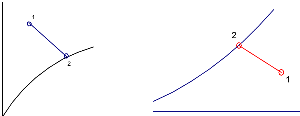
Figura 123: Rappresentazione della saturazione adiabatica dell'aria umida
