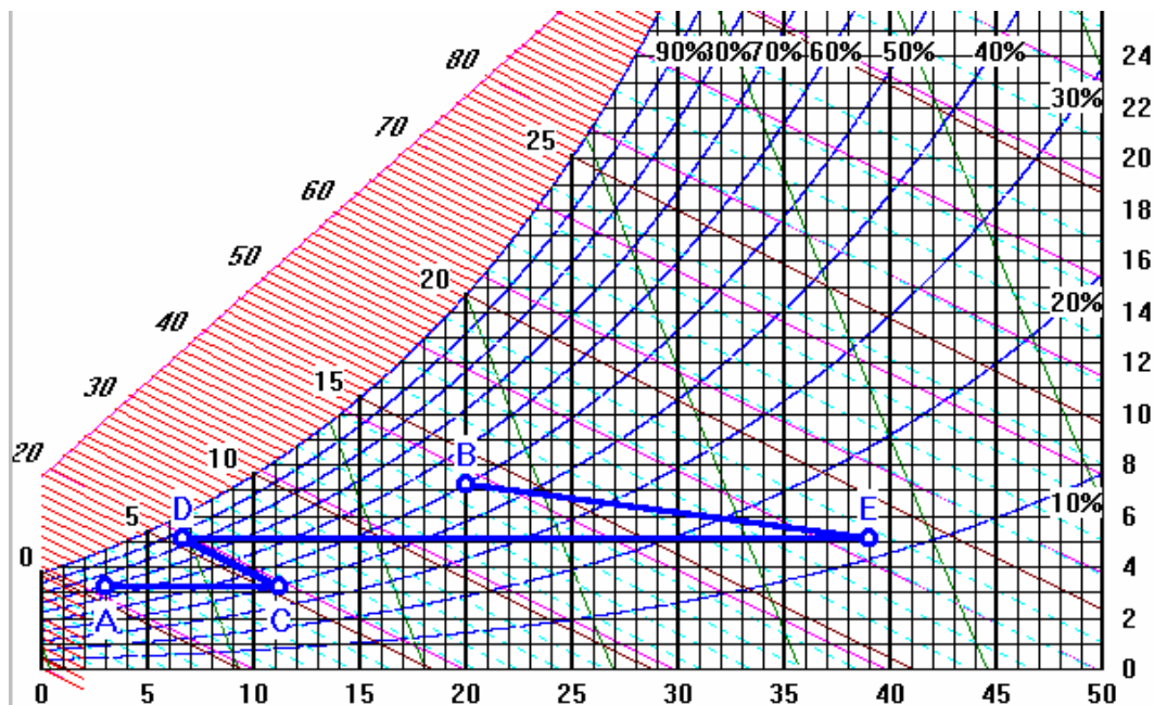
Figura 250: Ciclo di condizionamento invernale senza ricircolo nel piano ASHRAE
