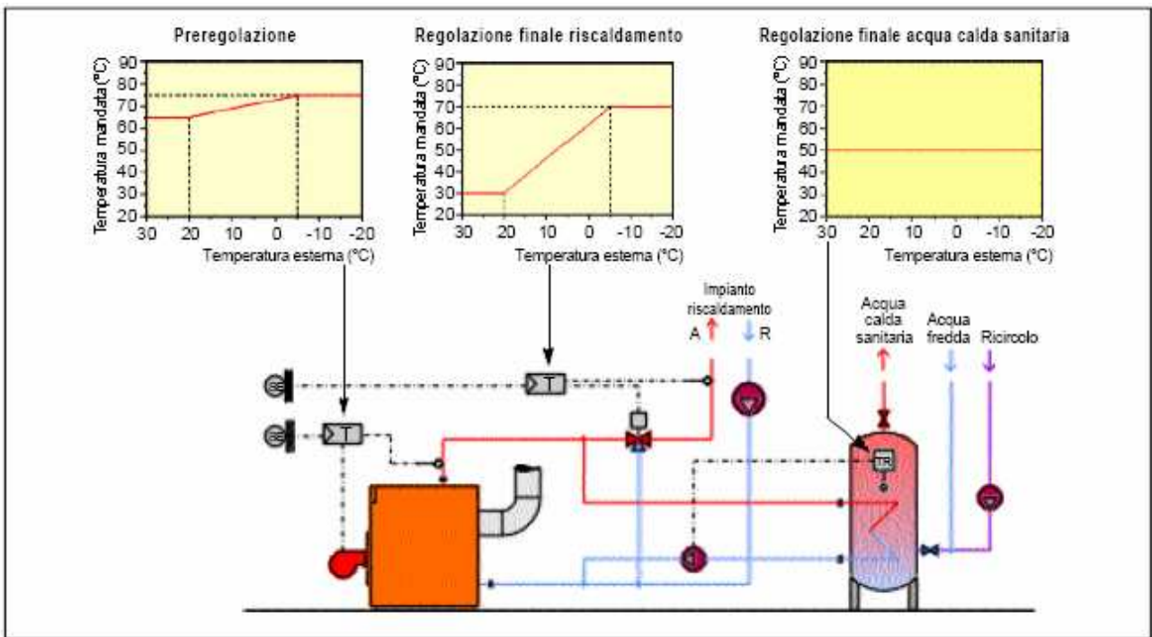
Figura 164: Generatore combinato per riscaldamento e acqua sanitaria
