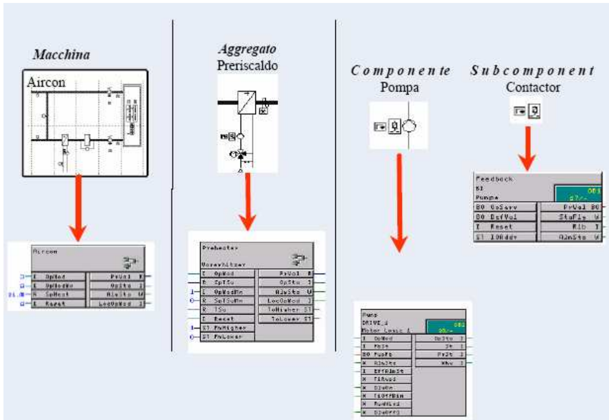
Figura 325: Esempi di programmazione dei controller locali : librerie di sottoprogrammi
