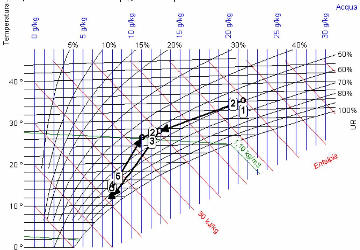
Figura 248: Ciclo estivo con ricircolo e postriscaldamento nel piano di Mollier
