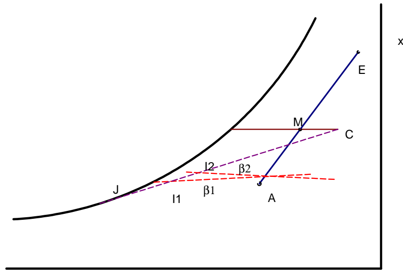
Figura 257: Trasformazioni per dual conduit in regime estivo
