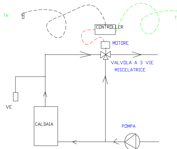
Figura 309: Sistema di controllo con sonda esterna ed interna
