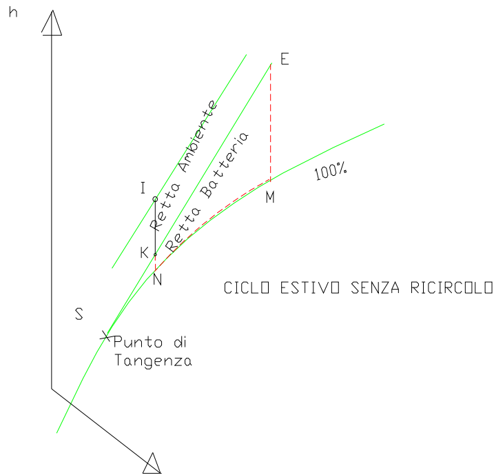
Figura 234: Ciclo estivo senza ricircolo con postriscaldamento
