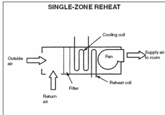
Figura 351: Controllo mediante post riscaldamento
