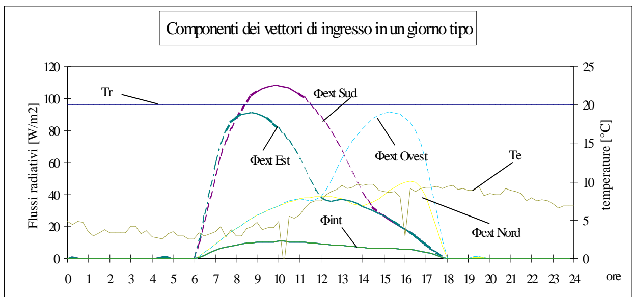
Figura 50: Andamento delle radiazioni per varie esposizioni
