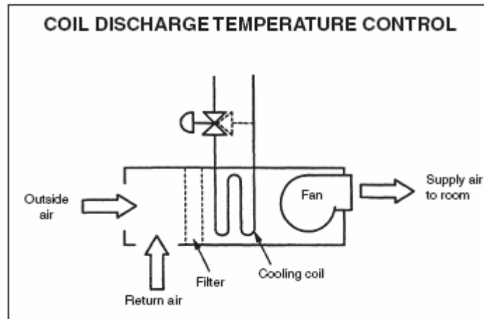
Figura 350: Sistema di controllo della temperatura della batteria
