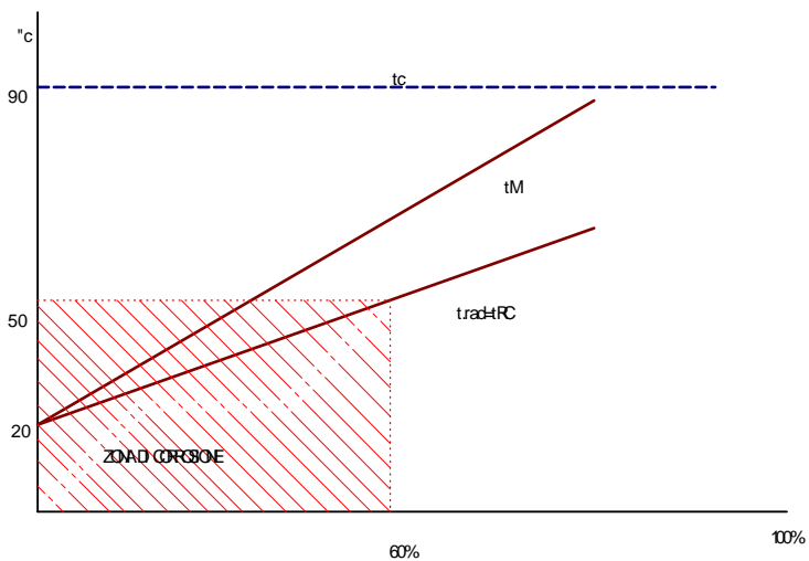
Figura 335: Andamento delle temperature nella zona di corrosione
