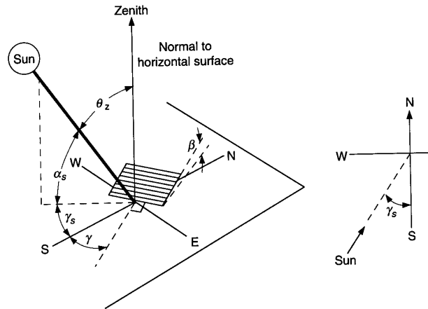
Figura 207: Definizioni degli angoli solari
