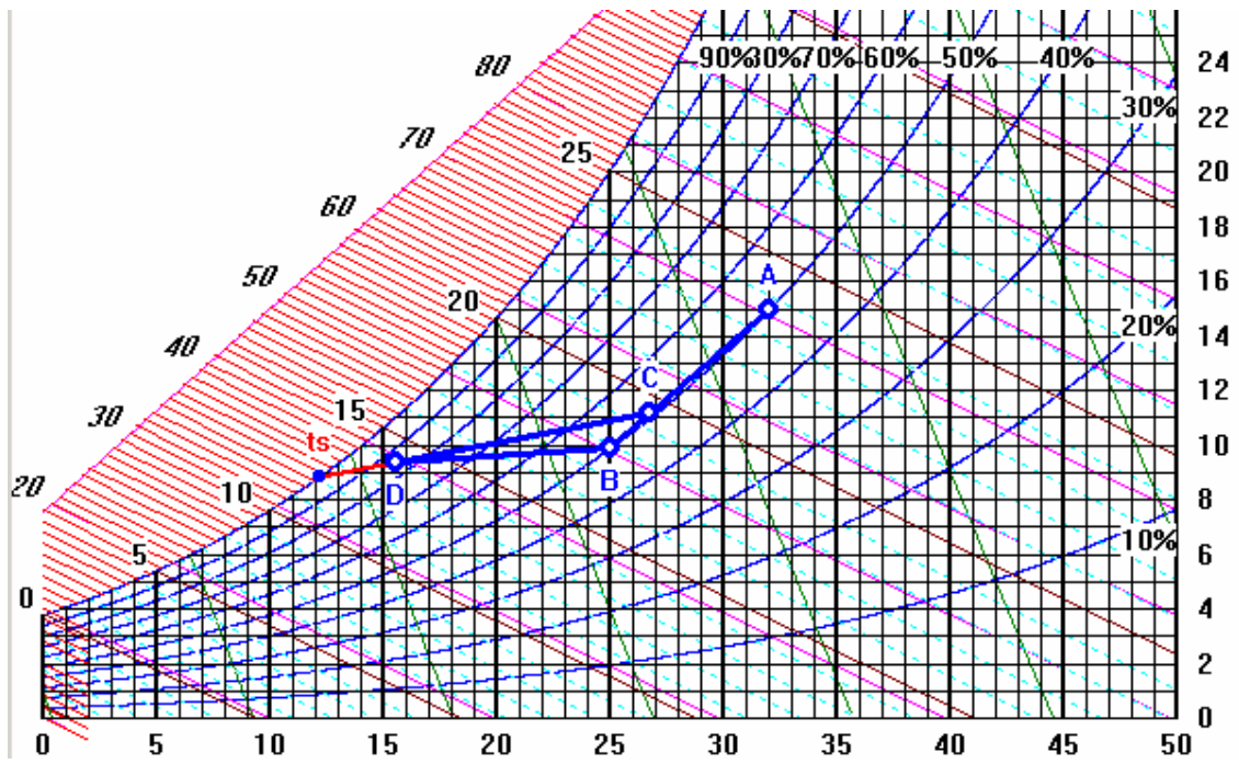
Figura 134: Esempio di climatizzazione estiva nel piano Asbrae - Carrier
