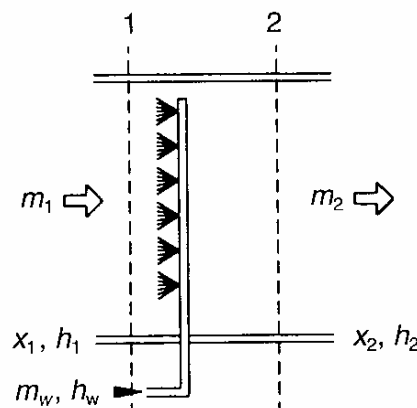
Figura 220: Schema di umidificazione adiabatica con liquido
