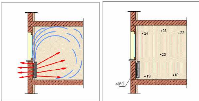
Figura 155: Esempio di disuniformità nella distribuzione del calore negli ambienti
