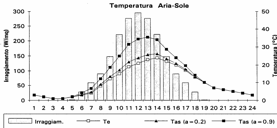
Figura 35: Andamento della temperatura aria-sole per a=0.2 e a=0.9 per un dato irraggiamento.
