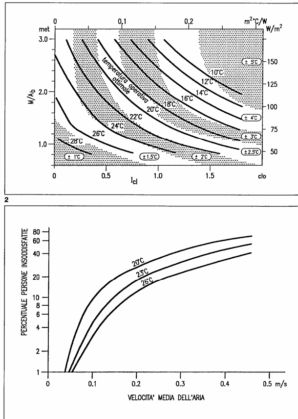
Figura 12: Condizioni di benessere ( M/A_D , I_{cl} ) e della PPD al variare della velocità media dell'aria.
