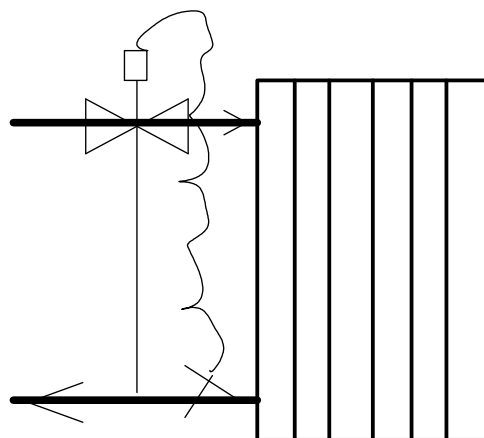
Figura 340: Valvola termostatica con controllo sul ritorno
