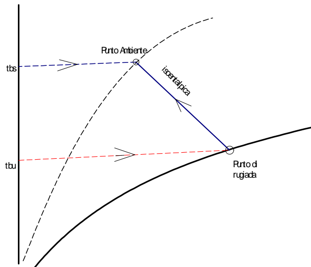
Figura 125: Determinazione del punto ambiente mediante uno psicrometro
