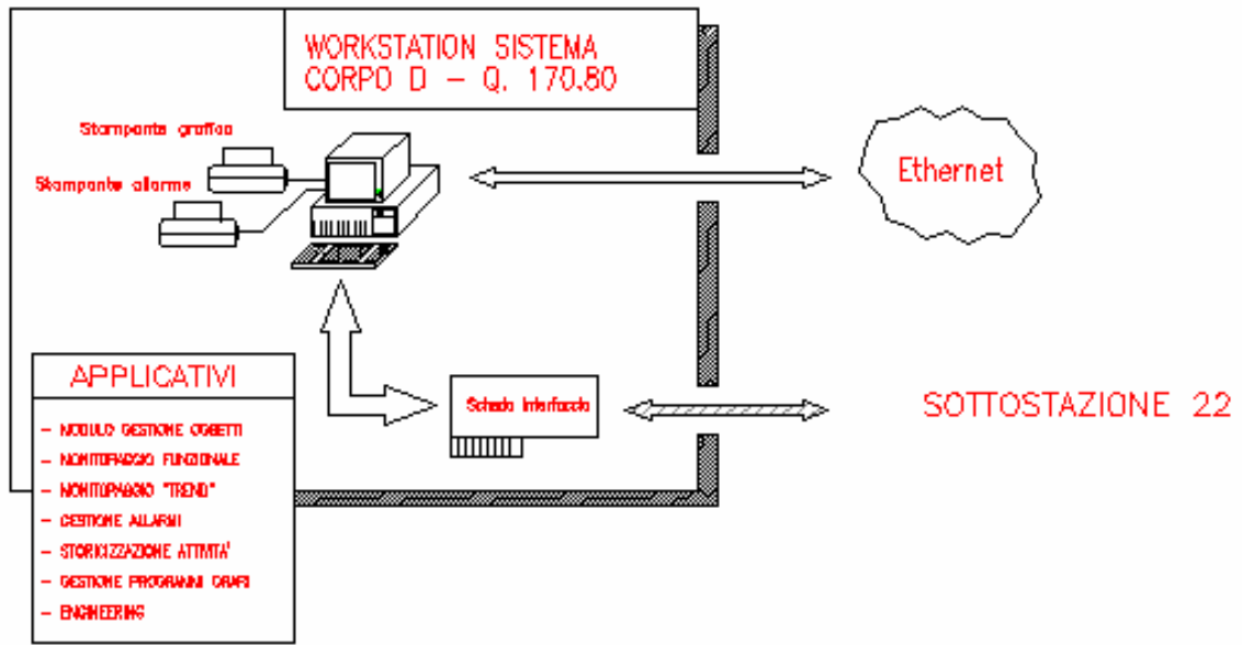
Figura 323: Layout del controller principale di impianto
