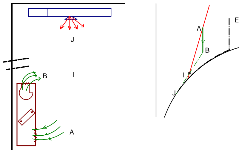
Figura 265: Schema di funzionamento di un fan coil in regime estivo
