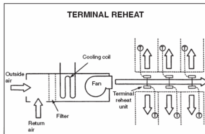
Figura 352: Controllo con post riscaldamento in impianto multizona
