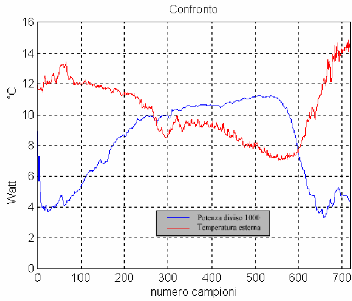
Figura 292: Andamento della temperatura esterna nel sistema studiato e della potenza ceduta
