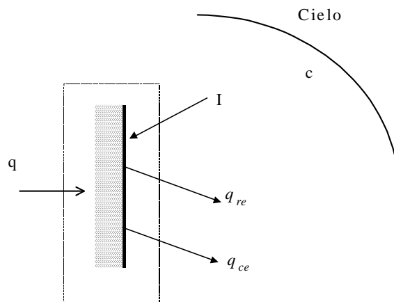
Figura 34: Scambi termici di una parete esterna soleggiata.
