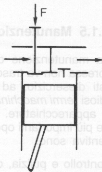
Fig. CP1.49 - Regolazione per apertura della valvola d'aspirazione.
