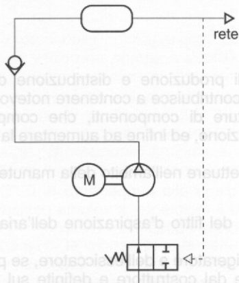
Fig. CP1.48 - Regolazione per chiusura dell'aspirazione.
