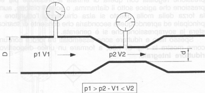
Fig. CP1.40 - Principio di Venturi.
