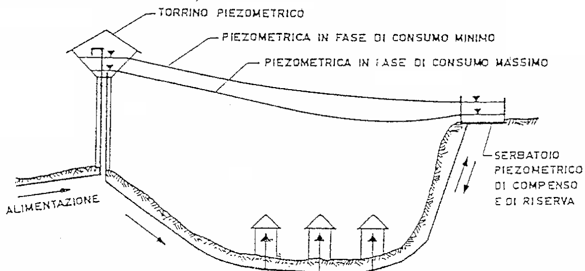
c) Schema con alimentazione diretta in rete da un impianto di sollevamento (Figura 3.3).
