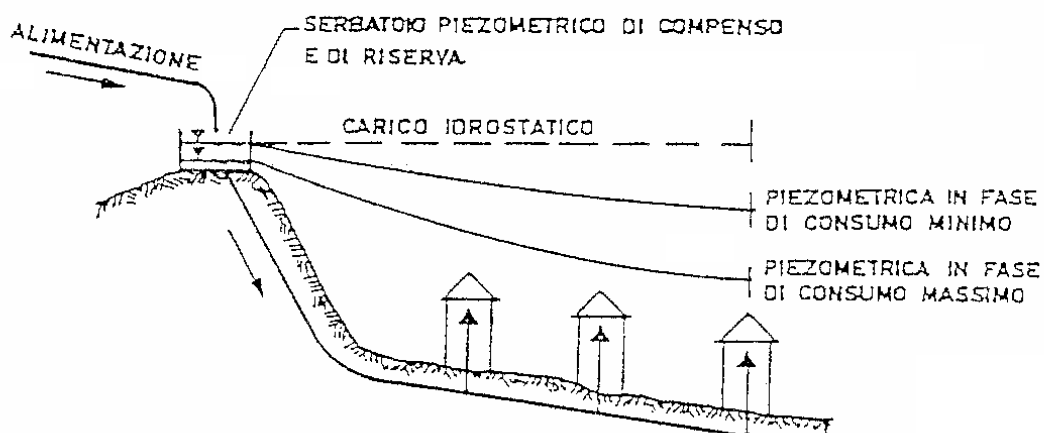
Figura 3.2 - Schema con due serbatoi, di testata e d'estremità.
