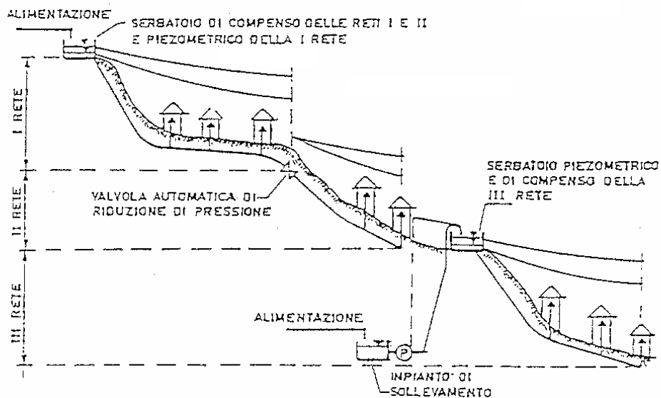
Figura 3.5 - Schema con un serbatoio unico per le due reti alte e un serbatoio per la terza rete
