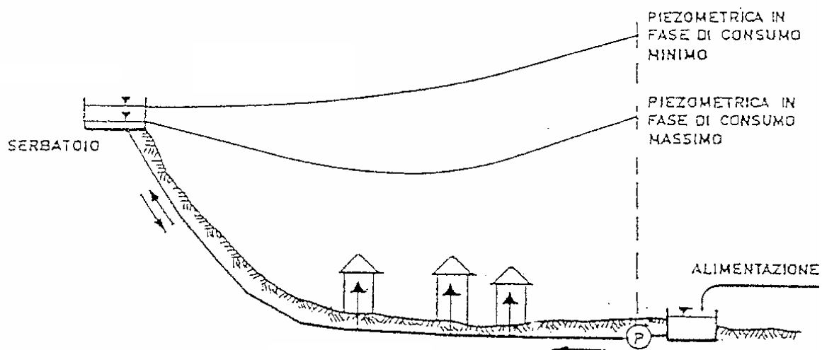
Figura 3.3 - Schema con alimentazione diretta in rete da un impianto di sollevamento.
